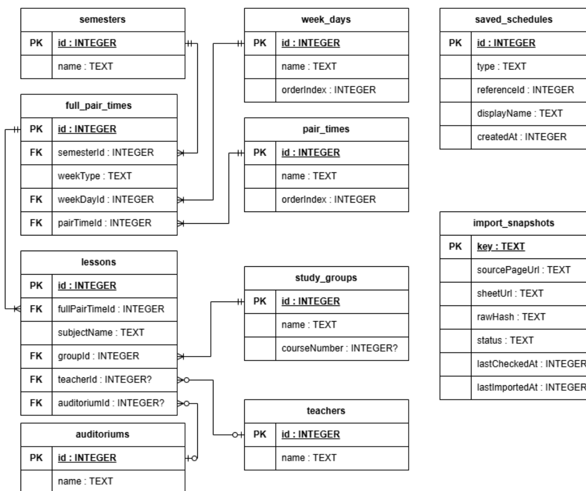
Рисунок 10 - ER-диаграмма базы данных
