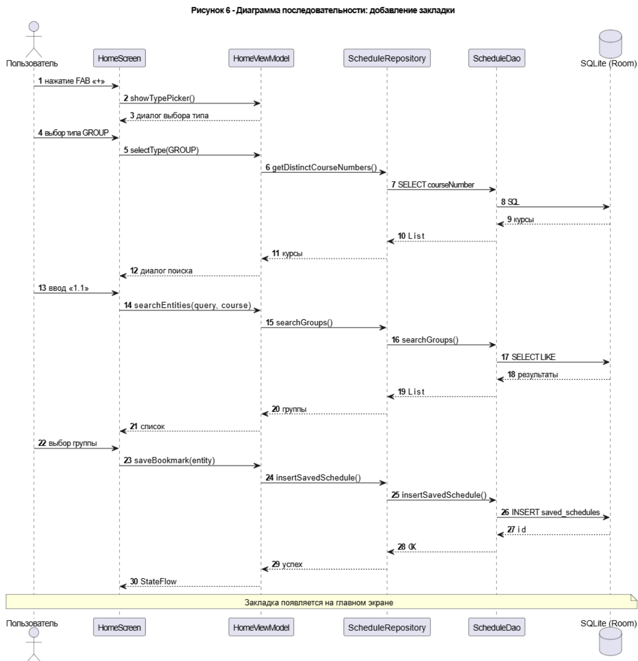
Рисунок 6 - Диаграмма последовательности: добавление закладки
