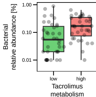
Roseburia
