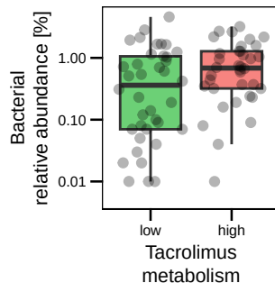
Dorea
