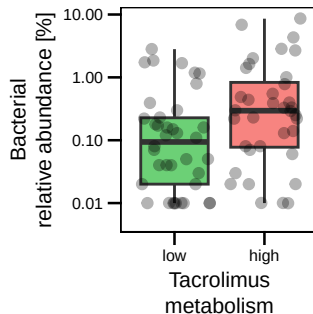
Lachnospiraceae
