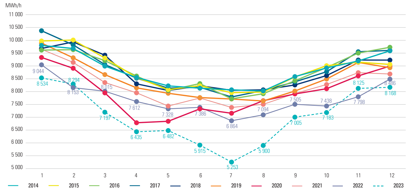
Figuur 10: Gemiddelde belasting op maandbasis op het Elia-net van 2014 tot 2023 (Bronnen: gegevens Elia, berekeningen CREG)
