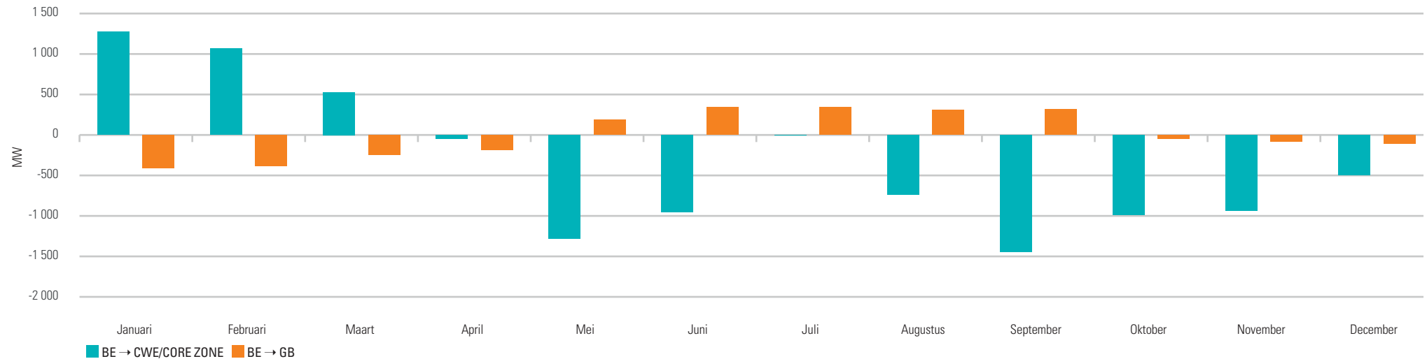
Figuur 4: Maandelijkse gemiddelden van de dagelijkse grensoverschrijdende uitwisselingen van België in de CWE/Core-regio en naar Groot-Brittannië in 2023, inclusief nominaties op lange termijn. Een positieve waarde wijst op een netto-uitvoer (> 0) en een negatieve waarde op een netto-invoer (< 0) (Bronnen: TNB's CWE, ENTSO-E Transparency platform, berekeningen CREG)
