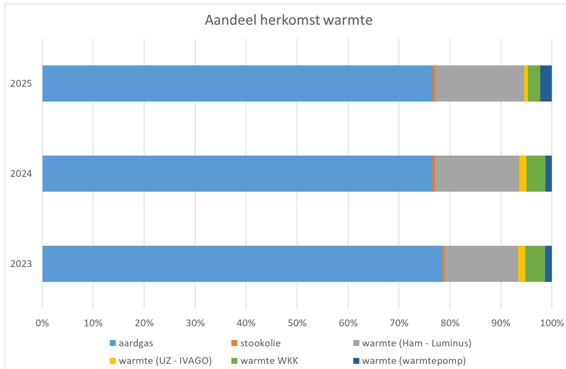
Figuur 3 : aandeel herkomst warmte 2023 -2025
