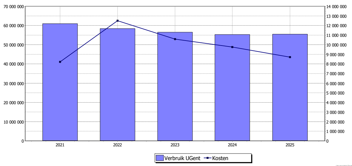
Figuur 6 : evolutie van het elektriciteitsverbruik en –kosten 2021 -2025
