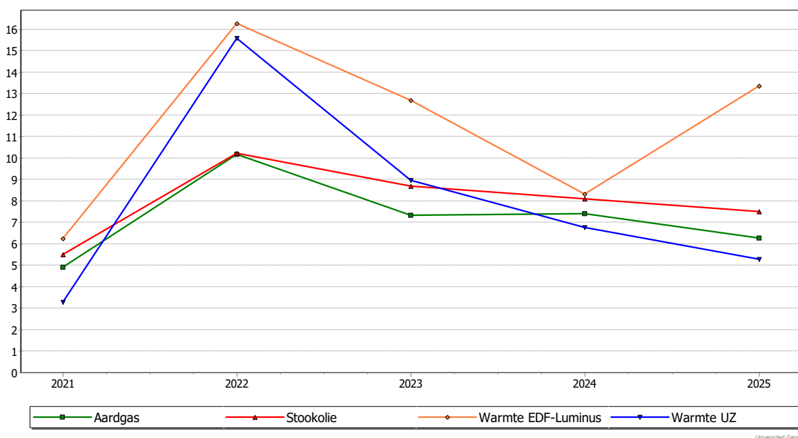
Figuur 4 : evolutie van de specifieke brandstof kosten: 2021 -2025
