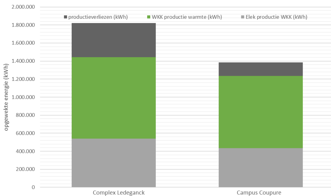
Figuur 9 : overzicht van de energiestromen van de WKK's op Ledeganck en Coupure in 2025
