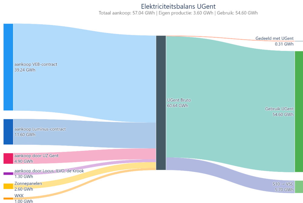
Figuur 11 : Sankey diagram van de elektriciteitsaankopen en gebruiken van UGent van 2025
