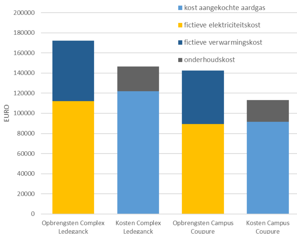
Figuur 10 : fictieve en werkelijke kosten van de WKK's
