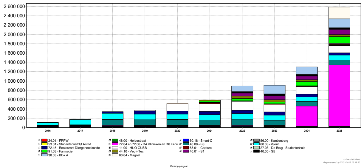
Figuur 7 : Overzicht van de elektriciteitsproductie van de PV-installaties (2016 - 2025)
