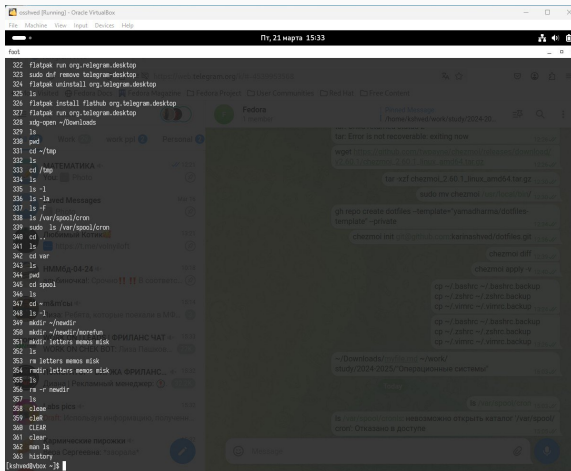
Рис. 11: history
