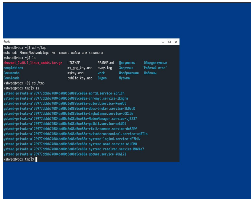
Рис. 2: стандартный вывод
