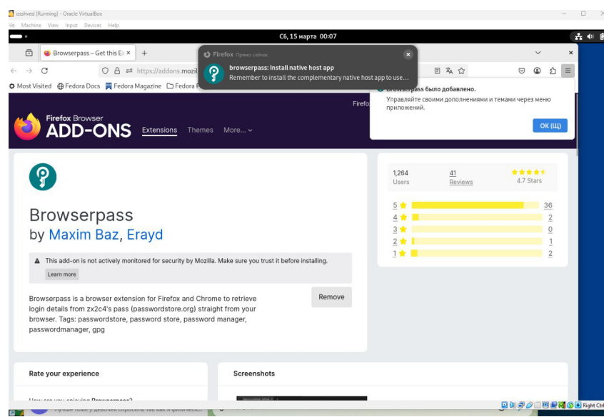
Рис. 5: настройка Browserpass
