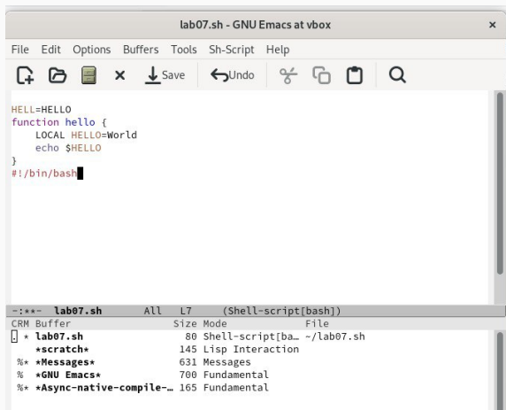
Рис. 4: список активных буферов
