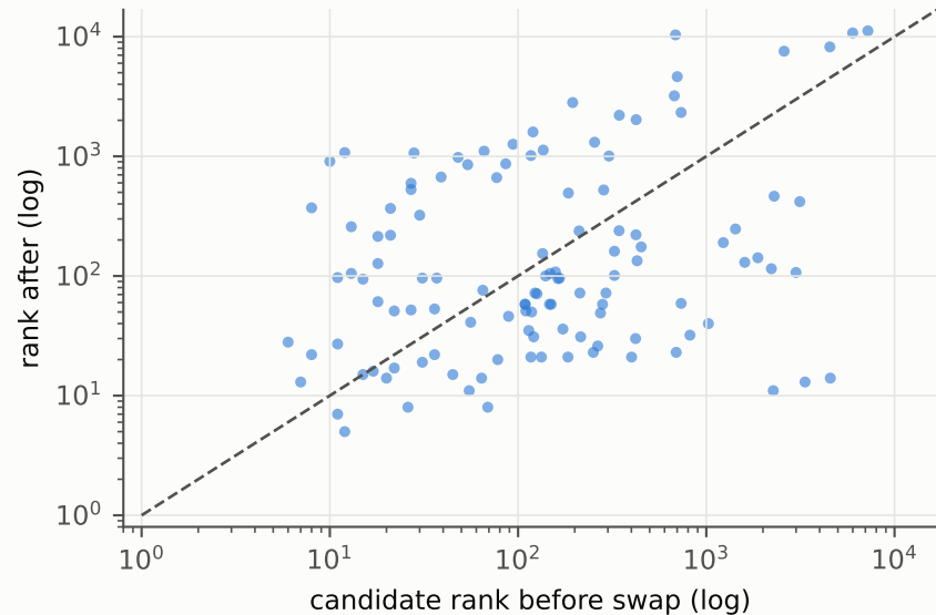
rank shift per trial (n=118; 64 improved, 54 not)
