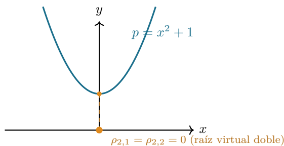
Figure 1: Raíces que siempre están ahí. El polinomio x^2 + 1 no tiene raíz real, pero sí una raíz virtual doble en x = 0 , donde la gráfica más se acerca al eje. Un polinomio de grado 2 tiene dos raíces virtuales sea cual sea su discriminante; aquí coinciden. En Lean, sobre un intervalo de encuadre, la construcción devuelve la lista [0, 0] .
