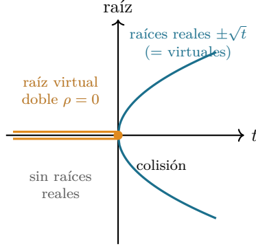
Figure 4: Raíces que siempre están ahí, al mover un parámetro. Para p_t = x^2 - t las dos raíces reales \pm\sqrt{t} (teal) existen solo para t \geq 0 y desaparecen al caer t por debajo de 0; las dos raíces virtuales (ámbar) persisten para todo t , coincidiendo con las reales cuando t \geq 0 y colisionando en la raíz virtual doble \rho = 0 para t < 0 . El recuento de raíces reales salta 2 \rightarrow 0 en t = 0 ; el de virtuales se queda en 2. La colisión en t = 0 es exactamente donde se forma un par conjugado—el origen del excedente par de Budan–Fourier. (Otra vista del mismo fenómeno que la Figura 1, ahora en movimiento.)
