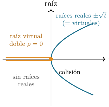
Figure 4: Raíces que siempre están ahí, al mover un parámetro. Para p_t = x^2 - t las dos raíces reales \pm\sqrt{t} (teal) existen solo para t \geq 0 y desaparecen al caer t por debajo de 0; las dos raíces virtuales (ámbar) persisten para todo t , coincidiendo con las reales cuando t \geq 0 y colisionando en la raíz virtual doble \rho = 0 para t < 0 . El recuento de raíces reales salta 2 \rightarrow 0 en t = 0 ; el de virtuales se queda en 2. La colisión en t = 0 es exactamente donde se forma un par conjugado—el origen del excedente par de Budan–Fourier. (Otra vista del mismo fenómeno que la Figura 1, ahora en movimiento.)
