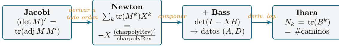
Figura 1: La columna vertebral del artículo. Un hecho elemental—la derivada de un determinante es una traza (Jacobi)—, llevado a todos los órdenes, se vuelve el diccionario entre las trazas de una matriz y su polinomio característico (Newton), y compuesto con la fórmula del determinante de Bass alcanza los conteos de caminos cerrados sin retroceso N_k = \text{tr}(B^k) de un grafo. Cada flecha es un teorema de este artículo.
