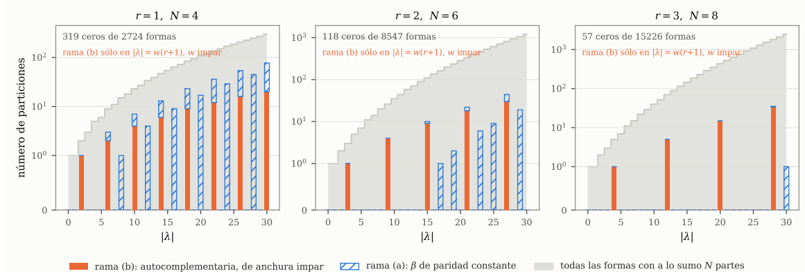
Figura 12. El lugar de anulación del Teorema 8.1, contado en lugar de dibujado. Para cada tamaño |\lambda| las barras dan el número de particiones con a lo sumo N partes que se anulan, separadas por rama; el escalón sombreado es el número total de formas de ese tamaño, en el mismo eje, de modo que la rareza del lugar se ve y no se afirma. Los tamaños que llevan la rama (b) son exactamente los múltiplos w(r+1) con w impar, por el Corolario 8.2; la rama (a) ocupa otros tamaños y necesita que el conjunto beta se salte una paridad por completo, razón por la cual está ausente en |\lambda| pequeño en cuanto N crece.
