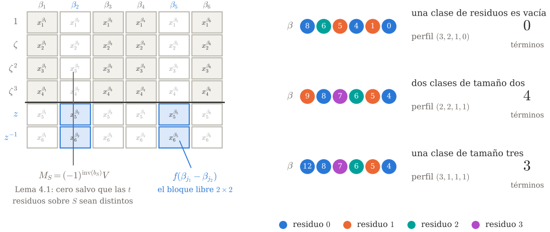
Figura 8. La arquitectura de la demostración, dibujada con t = 4 , N = 6 . Izquierda: el determinante \det(x_i^{\beta_j}) desarrollado por las t filas congeladas. Cada elección de las dos columnas U = \{j_1 < j_2\} que se dejan a las filas libres z, z^{-1} deja un menor t \times t M_S sobre las columnas complementarias, que por el Lema 4.1 vale \pm V o cero, por el bloque 2 \times 2 f(\beta_{j_1} - \beta_{j_2}) . Derecha: por el recuento del exceso dos (3) sólo hay tres perfiles de residuos, uno por fila, cada uno sobre un beta-conjunto que lo realiza; el número de la derecha es cuántas elecciones de U sobreviven, contado y no afirmado — 0, 4 y 3, que es la tricotomía sobre la que se organiza la sección. El color es la clase de residuos. Calculada por anc/fig_proof.py .
