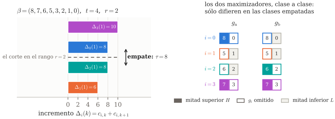
Figura 16. El Teorema 8.17 hecho sobre una forma, en vez de enunciado. Para \beta = (8, 7, 6, 5, 3, 2, 1, 0) con t = 4 , r = 2 las cuatro clases de exceso son \{8, 0\} , \{5, 1\} , \{6, 2\} , \{7, 3\} y los cuatro incrementos son \Delta_3(1) = 10 , \Delta_0(1) = 8 , \Delta_2(1) = 8 , \Delta_1(1) = 6 . Un maximizador toma los r = 2 mayores; el segundo y el tercero son iguales, así que \tau = \Delta_{(2)} = \Delta_{(3)} = 8 y hay exactamente dos. La pareja empatada pertenece a las clases 0 y 2 = 0 + t/2 , que es (34) y no una casualidad: ningún valor lo comparten incrementos de clases distintas de i e i + t/2 . A la derecha los dos maximizadores están dibujados clase a clase en la forma de prefijo del Paso 2 — leyendo una clase en orden decreciente, primero los elementos de la mitad de arriba, luego el omitido g_i , luego los de la mitad de abajo —, lo que hace visible que difieren en las clases empatadas y en ninguna otra. El color codifica la clase, no el rango. Calculada por anc/fig_v2.py .
