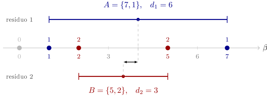
Figura 5. El mecanismo para t = 3 , \lambda = (3, 2) : aquí N = 5 , \beta = (7, 5, 2, 1, 0) con residuos (1, 2, 2, 1, 0) módulo 3, de modo que ninguna clase es vacía y dos clases tienen tamaño dos. Los tres argumentos de (5) son las dos longitudes de los intervalos y el doble de la distancia entre sus centros; la flecha doble corta marca esa distancia, aquí \frac{1}{2} , de modo que d_3 = 1 .
