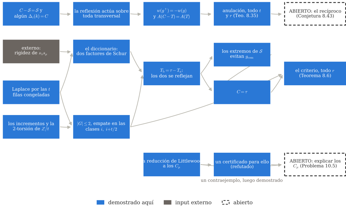
Figura 20. Sobre qué se apoya el criterio de la §8 y qué queda. Las cajas son enunciados y las flechas dependencias; el color es la columna de estado de la §9 —relleno lo demostrado aquí, gris el único apoyo ajeno, discontinuo lo abierto. La rama de arriba es el argumento extremal de las §§8.5 y 8.6; la de abajo es la reducción de Littlewood, cuyo certificado refuta la Proposición 8.11 —un contraejemplo, o sea una demostración—, de modo que la rama de abajo ya no toca el criterio sino la cuestión aparte de explicar los C_\mu , que es el Problema 10.5. Los enunciados van por nombre y no por número, para que la figura no pueda desfasarse cuando la numeración lo haga. Calculada por anc/fig_proof.py .
