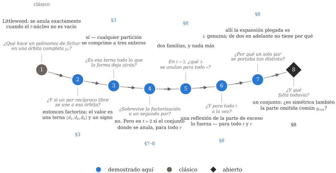
Figura 1. El artículo como un solo hilo. Cada pregunta la responde la perla que tiene debajo, y cada respuesta es lo que hace que la siguiente pregunta sea la natural: la órbita pide el par libre, la factorización pide la terna, la terna pide el segundo par, y el segundo par convierte una fórmula en un lugar. El color distingue lo clásico, lo demostrado aquí y lo que queda abierto, y la etiqueta bajo cada respuesta es la sección que la resuelve. Dibujada por anc/fig_intro.py .
