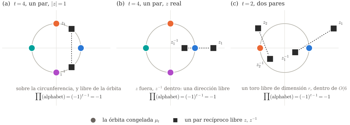
Figura 2. El alfabeto, en el plano complejo. La órbita \mu_t está congelada —un t -gono regular sobre la circunferencia unidad, coloreado por residuo— y cada par recíproco es una dirección compleja libre, dibujada unida por un segmento discontinuo. (a) el par puede estar sobre la circunferencia; es una variable libre y no parte de la órbita, y salvo para finitos z no toca \mu_t , que es la razón de que un operador hecho para órbitas de \zeta no tenga nada que decir de él. (b) fuera de la circunferencia, z por fuera y z^{-1} por dentro. (c) r pares dan un toro libre de dimensión r . En todos los casos el alfabeto es cerrado por inversión, así que es la lista de valores propios de un elemento de O(N, \mathbb{C}) —el panel (b) muestra por qué el grupo tiene que ser el complejo— y el producto de sus letras vale \zeta^{t(t-1)/2} = (-1)^{t-1} : para t par esa matriz está en la componente no identidad. Calculada por anc/fig_intro.py .
