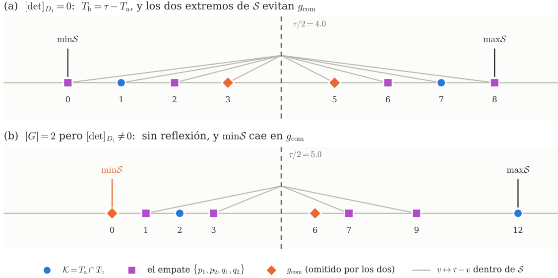
Figura 17. El Corolario 8.30 y la Proposición 8.32 sobre dos formas, las dos con t = 4 , r = 2 y |G| = 2 . Cada panel dibuja \mathcal{S} sobre una recta, coloreada según a qué parte de (38) pertenece el valor; un arco une v con \tau - v cuando los dos están en \mathcal{S} , y la línea discontinua es el centro \tau/2 . (a) \beta = (8, 7, 6, 5, 3, 2, 1, 0) : \tau = 8 , \mathcal{K} = \{1, 7\} , g_{\text{com}} = \{3, 5\} , empate \{0, 2, 6, 8\} . Aquí T_b = \tau - T_a , así que \mathcal{S} \setminus g_{\text{com}} es simétrico respecto de \tau/2 , y los dos extremos de \mathcal{S} evitan g_{\text{com}} , luego C = 0 + 8 = \tau . Aquí g_{\text{com}} = \{3, 5\} resulta ser simétrico también —el arco que une sus dos miembros se dibuja como cualquier otro—, que es lo que la Conjetura 8.44 afirma en general y lo que la §8.6 no demuestra: la reflexión queda establecida sobre \mathcal{S} \setminus g_{\text{com}} y observada en el resto. (b) \beta = (12, 9, 7, 6, 3, 2, 1, 0) : aquí \tau = 10 , y otra vez |G| = 2 , pero los dos maximizadores no son reflexión uno de otro; \min \mathcal{S} = 0 cae en g_{\text{com}} , y C = 0 + 12 = 12 \neq \tau . El panel (b) es la razón de que la Proposición 8.32 no pueda demostrarse sólo a partir de |G| = 2 . Calculada por anc/fig_v2.py .
