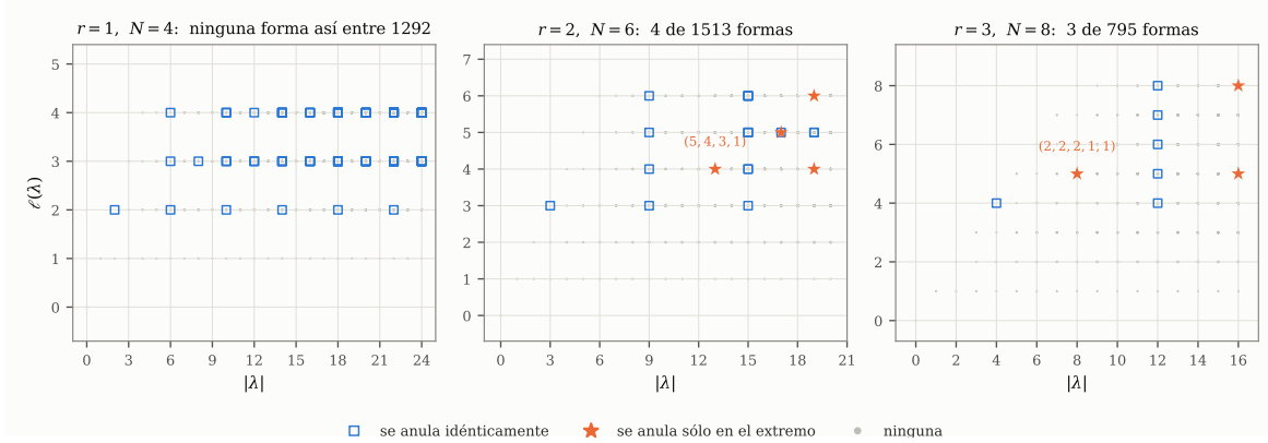
Figura 15. Dónde deja de ser típico un solo par recíproco. Cada partición con a lo sumo N partes es un punto en (|\lambda|, \ell(\lambda)) ; la clase dibujada con estrella es la que se anula en el extremo z_i = 1 sin anularse idénticamente, y es todo el contenido de la imagen; cada panel nombra a su miembro más pequeño y la Observación 8.12 enumera los demás. Los paneles cubren |\lambda| \leq 24, 20 y 16 respectivamente. En r = 1 la clase está vacía sobre las 1292 formas del rango, porque allí el objeto es \pm un carácter genuino y su valor en la identidad es una dimensión. A partir de r = 2 aparecen ejemplos genuinamente virtuales y la clase deja de estar vacía —no que toda forma lo sea: el Cuadro 2 cuenta las dos cosas—. Véase la Observación 8.12.
