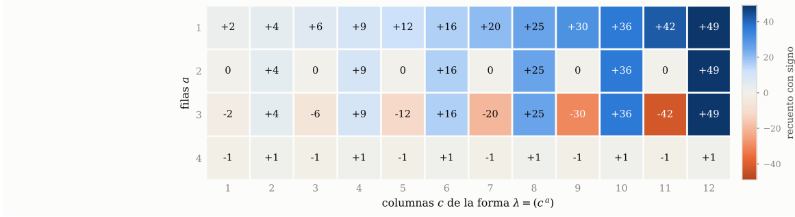
Figura 10. Los recuentos con signo del Ejemplo 6.2: el valor del Corolario 6.1 en z = 1 y t = 2 para las formas rectangulares \lambda = (c^a) , esto es la (-1) -enumeración de particiones planas en una caja a \times (4 - a) \times c . Cada entrada es la forma cerrada \varepsilon_\lambda d_1 d_2 d_3 / (2t^2) , contrastada contra una enumeración directa de las tablas. La fila a = 2 se anula para c impar y es un cuadrado perfecto para c par.
