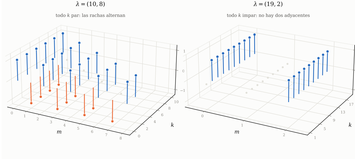
Figura 11. La Proposición 6.4, dibujada. Para cada k las \nu admisibles son la única familia (m+k, m) , y se representa \sigma_m = s_{\lambda/(m+k, m)}(1, -1) frente a m y k ; los puntos grises son los ceros. Toda barra tiene altura exactamente \pm 1 , que es la parte (i): los términos forman un conjunto, luego la cancelación que pide la enumeración es un emparejamiento y no algo con multiplicidad. A la izquierda todo k es par y el color alterna a lo largo de cada racha, que es la parte (iii) y lo que hace que m \leftrightarrow m+1 invierta el signo; donde una racha acaba, la acaba un cero. A la derecha todo k es impar y no hay dos términos no nulos contiguos, que es la parte (ii): las rachas tienen longitud uno y no hay nada que cancelar.
