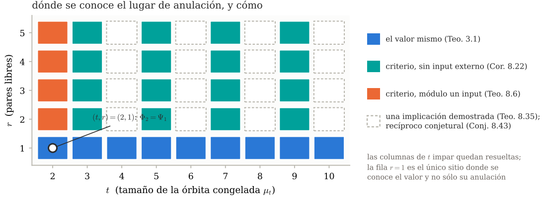
Figura 3. La familia de dos parámetros, y lo que se sabe sobre ella. Cada celda es un alfabeto \mu_t \cup \{z_1^{\pm 1}, \dots, z_r^{\pm 1}\} ; el color no se asigna a mano, sino que se calcula a partir de los propios enunciados, con una regla por línea del artículo. La fila r = 1 es el único sitio donde se conoce el valor y no sólo su anulación, que es el Teorema 3.1; las columnas de t impar las resuelve el Corolario 8.22 sin ningún input externo; la columna t = 2 , el Teorema 8.6, que usa uno. En las celdas restantes el Teorema 8.35 prueba una implicación y la Conjetura 8.43 es la otra. La esquina marcada es donde se encuentran las dos mitades del artículo: allí \Phi_2 = \Psi_1 , y es el único alfabeto que ven las dos. Calculada por anc/fig_plane.py .
