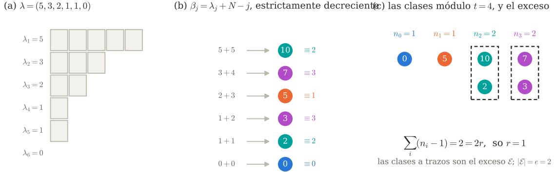
Figura 4. El diccionario sobre el que corre el resto del artículo, con \lambda = (5, 3, 2, 1, 1, 0) y t = 4 . (a) la forma, rellenada hasta N partes. (b) \beta_j = \lambda_j + N - j , que convierte una sucesión débilmente decreciente en una estrictamente decreciente y por tanto en un conjunto; cada valor se colorea después según su residuo módulo t . (c) el perfil de residuos (n_0, \dots, n_{t-1}) y el recuento (3): \sum_i (n_i - 1) = 2r siempre, de modo que cuando toda clase está ocupada las clases con n_i \geq 2 —el exceso \mathcal{E} , a trazos— llevan exactamente 2r elementos más de uno cada una. Si alguna está vacía la suma sigue valiendo 2r pero ya no es un exceso: ésa es la rama degenerada, que se resuelve la primera. Todo lo que el artículo demuestra es un enunciado sobre ese dibujo. Calculada por anc/fig_intro.py .
