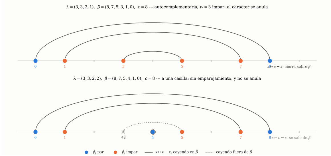
Figura 13. Por qué la autocomplementariedad mata el carácter. Al desarrollar por las dos filas congeladas quedan términos indexados por pares (e, o) con e \in E , o \in O , y la reflexión x \mapsto c - x actúa sobre ellos. Arriba, una forma autocomplementaria de anchura impar: todo arco cae dentro de \beta y une entradas de igual paridad, porque c es par. Abajo, la misma forma con una caja movida: el arco 5 \mapsto 3 se sale de \beta , así que no hay emparejamiento y nada se cancela. El rombo marca el punto fijo de la reflexión, que no puede darse dentro de un par de paridades opuestas —y ésa es la razón de que la involución sea libre.
