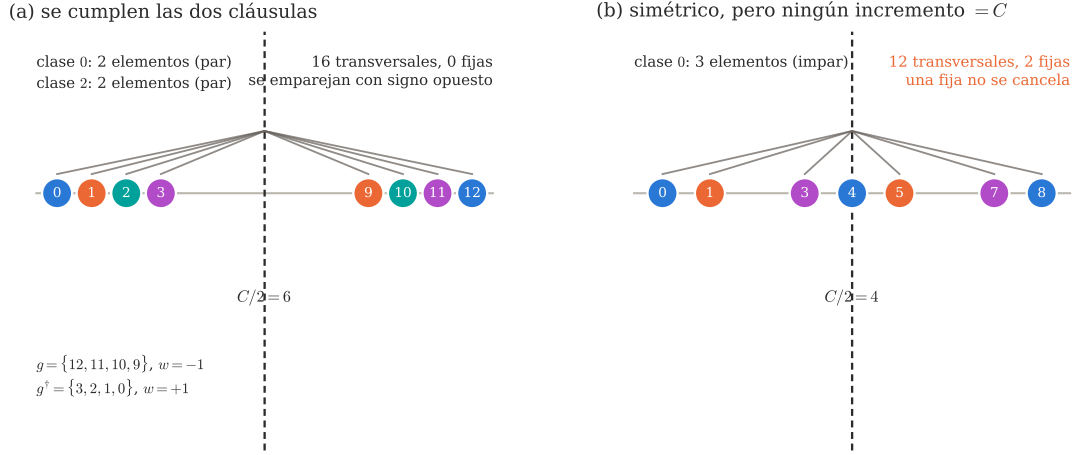
Figura 18. Por qué se cancela la suma, y para qué está la segunda cláusula. Cada panel dibuja \mathcal{S} sobre una recta, coloreado por clase de residuo, con un arco que une v con C - v y el eje de puntos en C/2 . (a) \beta = (12, 11, 10, 9, 3, 2, 1, 0) con t = 4 , r = 2 : las dos clases que la reflexión fija tienen tamaño par , así que ninguna contiene a C/2 ; las 16 transversales se emparejan sin ningún punto fijo, y cada pareja lleva signos opuestos, de modo que cada término de (28) lo cancela otro. Una de esas parejas está impresa con sus dos signos, calculados y no afirmados. (b) una forma con C - \mathcal{S} = \mathcal{S} pero sin ningún incremento igual a C , encontrada buscándola y no elegida: allí la clase fija tiene tamaño impar , luego contiene a C/2 , y dos transversales son su propio reflejo. Un término emparejado consigo mismo no puede cancelarse, y la suma sobrevive. Eso es todo lo que compra la segunda cláusula. Calculada por anc/fig_involution2.py .
