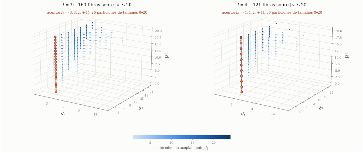
Figura 7. Las fibras del invariante de la evaluación (7), complemento de la Figura 6: el mismo rango |\lambda| \leq 20 , con el término de acoplamiento pasado al color y el tamaño |\lambda| en el eje vertical. Una columna es una fibra, así que su altura es el rango de tamaños que este alfabeto no sabe separar; las marcas del suelo son el retículo t\mathbb{Z} de la Proposición 3.4, y solo está ocupada la mitad d_1 \leq d_2 porque la terna se toma salvo el intercambio, como en la Figura 6. Que todas las marcas de una columna lleven el mismo valor está computado, no supuesto: sobre las 860 particiones de la izquierda y las 883 de la derecha el bialternante es constante en cada fibra hasta 10^{-37} . La columna en color de acento es la fibra de \lambda = \emptyset .
