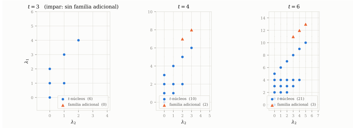
Figura 9. El Teorema 5.2, calculado y no afirmado. Para toda \lambda de dos filas en rango se evaluaron ambos miembros de \Phi_t(\lambda; z) = \pm s_\lambda(z, \bar{z}) ; se representan las particiones donde coinciden, coloreadas por familia. Los círculos son los t -núcleos, las soluciones ya descritas por (4); los triángulos son la familia adicional (17), que crea la especialización recíproca. El caso impar t=3 es el control: por el Teorema 5.2 allí no puede existir solución adicional, y no se halla ninguna.
