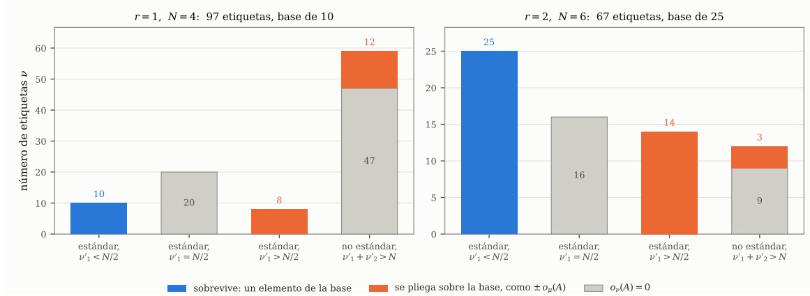
Figura 14. La reducción del Lema 8.9, dibujada. Cada etiqueta \nu que aparece en s_\lambda = \sum_\nu c_\nu o_\nu se coloca en una de cuatro clases y se calcula su valor o_\nu(A) . Las etiquetas autoasociadas se anulan, todas ellas; las estándar con \nu'_1 > N/2 se pliegan sobre la base como \pm o_\mu(A) ; las no estándar o se anulan o se pliegan sobre un único elemento de la base con coeficiente \pm 1 . Por (25) estas tres son las reglas de modificación simplécticas disfrazadas, con las clases cortadas por \ell(\nu) frente al rango r ; la figura se calculó antes de advertirlo y se deja tal cual. Todo aterriza en la base independiente \{o_\mu(A) : \ell(\mu) \leq r\} , que es lo que convierte la anulación en la condición finita (26). Las alturas de las barras son recuentos de etiquetas sobre el rango en que se calculó cada panel, menor que el de la fila correspondiente de la §9; lo que la imagen cuenta es la clasificación, no el recuento.
