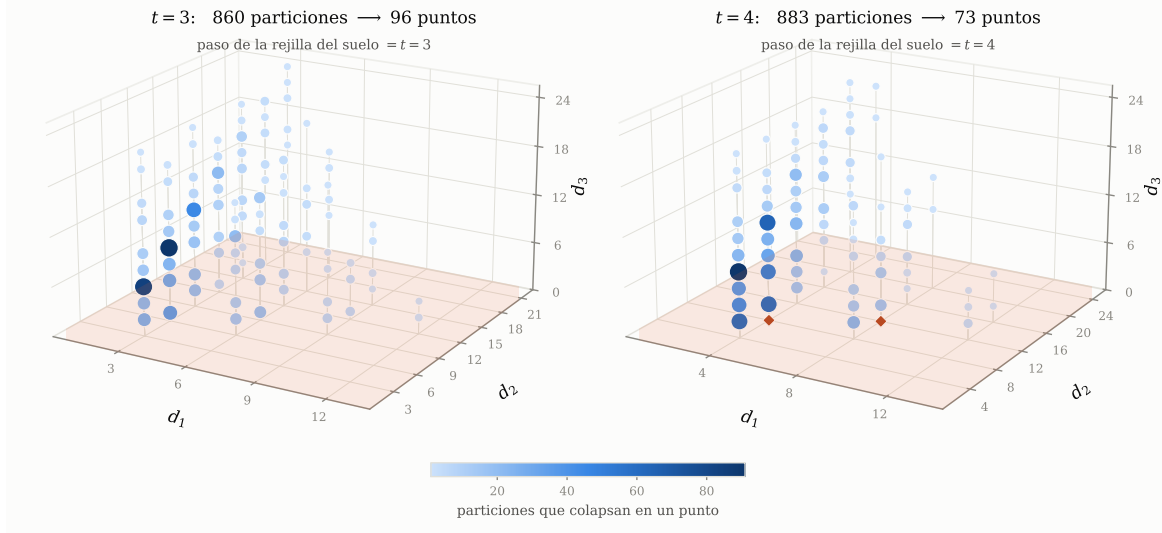
Figura 6. La imagen de \lambda \mapsto (d_1, d_2, d_3) sobre todas las \lambda con |\lambda| \leq 20 y a lo sumo t + 2 filas, para t = 3 (izquierda) y t = 4 (derecha), tomada salvo el intercambio de d_1 y d_2 , bajo el cual (5) es simétrica; sin esa identificación, y con A y B en el orden r_A \leq r_B del Teorema 3.1, los dos paneles llevan 126 y 92 puntos en vez de 96 y 73. La compresión es el asunto de la figura: 860 particiones aterrizan sobre 96 ternas a la izquierda y 883 sobre 73 a la derecha, y el color y el área dan el número de particiones que va a parar a cada una. El paso de la rejilla del suelo es t , pues d_1, d_2 \in t\mathbb{Z} por la Proposición 3.4; el plano sombreado d_3 = 0 es el lugar concéntrico del Corolario 3.2, donde s_\lambda se anula, así que esas formas no están en la imagen y se dibujan sobre el plano como rombos. Los dos paneles son las dos paridades, que es el contenido de la Proposición 3.5: el impar no lleva ningún rombo, y no puede llevarlo; el par lleva dos, que son entre ambos la imagen de 32 particiones.
