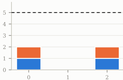
A_{16}(99), p=3: d=5, e=3 not Gorenstein
