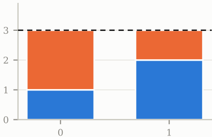
A_6(56), p=2: d=3, e=2 not Gorenstein
