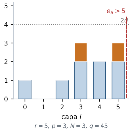
(c) p \mid N , desplazamiento 3
