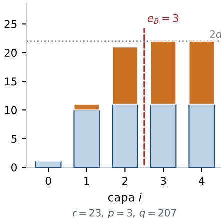
(b) \delta = 1 , desplazamiento 1
