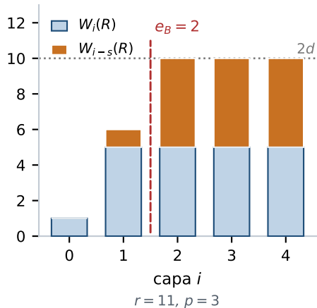
(a) \delta = 0 , desplazamiento 1
