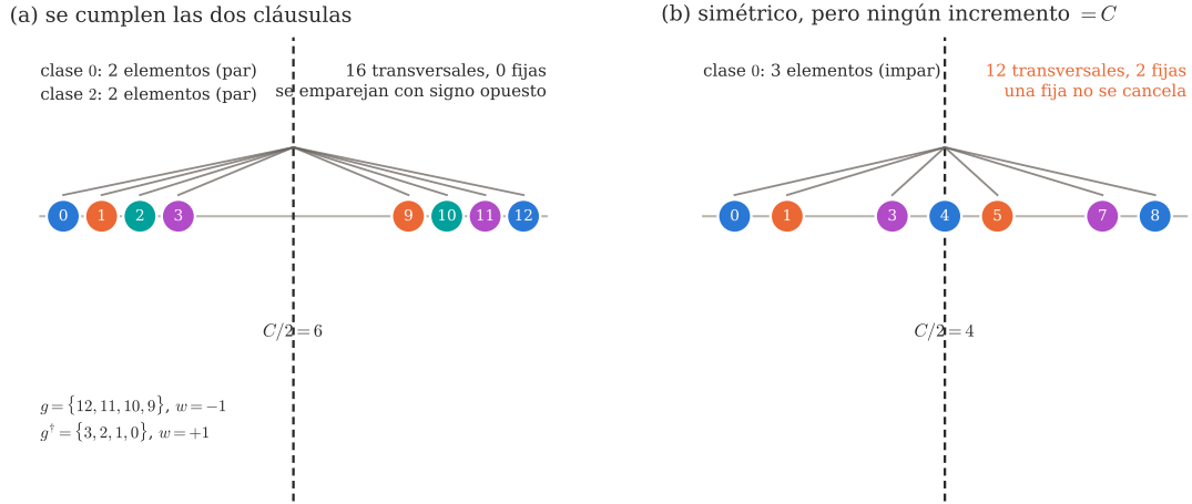
Figura 19. Por qué se cancela la suma, y para qué está la segunda cláusula. Cada panel dibuja \mathcal{S} sobre una recta, coloreado por clase de residuo, con un arco que une v con C - v y el eje de puntos en C/2 . (a) \beta = (12, 11, 10, 9, 3, 2, 1, 0) con t = 4 , r = 2 : las dos clases que la reflexión fija tienen tamaño par , así que ninguna contiene a C/2 ; las 16 transversales se emparejan sin ningún punto fijo, y cada pareja lleva signos opuestos, de modo que cada término de (29) lo cancela otro. Una de esas parejas está impresa con sus dos signos, calculados y no afirmados. (b) una forma con C - \mathcal{S} = \mathcal{S} pero sin ningún incremento igual a C , encontrada buscándola y no elegida: allí la clase fija tiene tamaño impar , luego contiene a C/2 , y dos transversales son su propio reflejo. Un término emparejado consigo mismo no puede cancelarse, y la suma sobrevive. Eso es todo lo que compra la segunda cláusula. Calculada por anc/fig_involution2.py .
