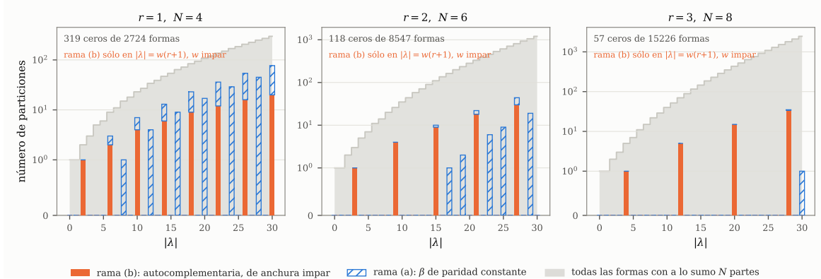
Figura 13. El lugar de anulación del Teorema 8.1, contado en lugar de dibujado. Para cada tamaño |\lambda| las barras dan el número de particiones con a lo sumo N partes que se anulan, separadas por rama; el escalón sombreado es el número total de formas de ese tamaño, en el mismo eje, de modo que la rareza del lugar se ve y no se afirma. Los tamaños que llevan la rama (b) son exactamente los múltiplos w(r+1) con w impar, por el Corolario 8.2; la rama (a) ocupa otros tamaños y necesita que el conjunto beta se salte una paridad por completo, razón por la cual está ausente en |\lambda| pequeño en cuanto N crece.
