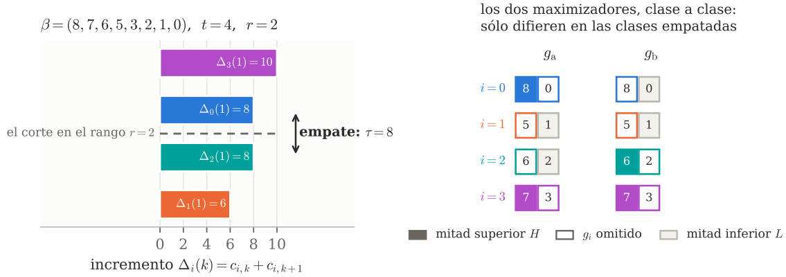
Figura 17. El Teorema 8.17 hecho sobre una forma, en vez de enunciado. Para \beta = (8, 7, 6, 5, 3, 2, 1, 0) con t = 4 , r = 2 las cuatro clases de exceso son \{8, 0\} , \{5, 1\} , \{6, 2\} , \{7, 3\} y los cuatro incrementos son \Delta_3(1) = 10 , \Delta_0(1) = 8 , \Delta_2(1) = 8 , \Delta_1(1) = 6 . Un maximizador toma los r = 2 mayores; el segundo y el tercero son iguales, así que \tau = \Delta_2 = \Delta_3 = 8 y hay exactamente dos. La pareja empatada pertenece a las clases 0 y 2 = 0 + t/2 , que es (35) y no una casualidad: ningún valor lo comparten incrementos de clases distintas de i e i + t/2 . A la derecha los dos maximizadores están dibujados clase a clase en la forma de prefijo del Paso 2 — leyendo una clase en orden decreciente, primero los elementos de la mitad de arriba, luego el omitido g_i , luego los de la mitad de abajo —, lo que hace visible que difieren en las clases empatadas y en ninguna otra. El color codifica la clase, no el rango. Calculada por anc/fig_v2.py .
