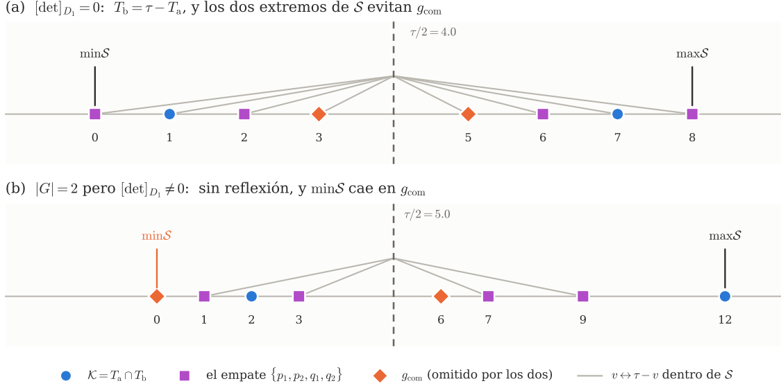
Figura 18. El Corolario 8.30 y la Proposición 8.32 sobre dos formas, las dos con t = 4 , r = 2 y |G| = 2 . Cada panel dibuja \mathcal{S} sobre una recta, coloreada según a qué parte de (39) pertenece el valor; un arco une v con \tau - v cuando los dos están en \mathcal{S} , y la línea discontinua es el centro \tau/2 . (a) \beta = (8, 7, 6, 5, 3, 2, 1, 0) : \tau = 8 , \mathcal{K} = \{1, 7\} , g_{\text{com}} = \{3, 5\} , empate \{0, 2, 6, 8\} . Aquí T_b = \tau - T_a , así que \mathcal{S} \setminus g_{\text{com}} es simétrico respecto de \tau/2 , y los dos extremos de \mathcal{S} evitan g_{\text{com}} , luego C = 0 + 8 = \tau . Aquí g_{\text{com}} = \{3, 5\} resulta ser simétrico también —el arco que une sus dos miembros se dibuja como cualquier otro—, que es lo que la Conjetura 8.44 afirma en general y lo que la §8.6 no demuestra: la reflexión queda establecida sobre \mathcal{S} \setminus g_{\text{com}} y observada en el resto. (b) \beta = (12, 9, 7, 6, 3, 2, 1, 0) : aquí \tau = 10 , y otra vez |G| = 2 , pero los dos maximizadores no son reflexión uno de otro; \min \mathcal{S} = 0 cae en g_{\text{com}} , y C = 0 + 12 = 12 \neq \tau . El panel (b) es la razón de que la Proposición 8.32 no pueda demostrarse sólo a partir de |G| = 2 . Calculada por anc/fig_v2.py .
