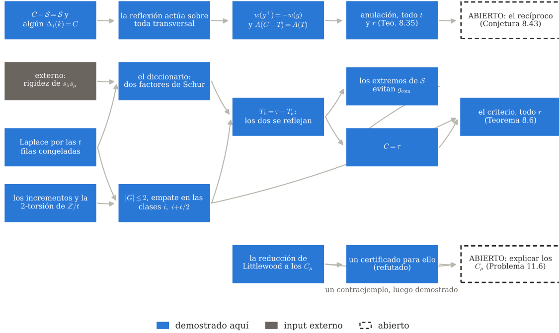
Figura 21. Sobre qué se apoya el criterio de la §8 y qué queda. Las cajas son enunciados y las flechas dependencias; el color es la columna de estado de la §9 —relleno lo demostrado aquí, gris el único apoyo ajeno, discontinuo lo abierto. La rama del medio es el argumento extremal de las §§8.5 y 8.6, que cierra el criterio en t = 2 para todo r . La de abajo es la reducción de Littlewood, cuyo certificado refuta la Proposición 8.11 —un contraejemplo, o sea una demostración—, de modo que ya no toca el criterio sino la cuestión aparte de explicar los C_\mu , que es el Problema 11.6. La de arriba arranca de una hipótesis y no del desarrollo, y es la única que alcanza todo t y todo r : allí la reflexión empareja todos los términos a la vez y no sólo los dos maximizadores. Las tres se encuentran en la única implicación que falta, que es lo que hace de la Conjetura 8.43 una conjetura. Las cajas nombran sus enunciados, y los cuatro números que sí llevan se leen del .aux al dibujar, de modo que no pueden desfasarse cuando la numeración lo haga; check_figrefs.py comprueba que cada uno sigue resolviendo, y a un enunciado del tipo correcto. Calculada por anc/fig_proof.py .
