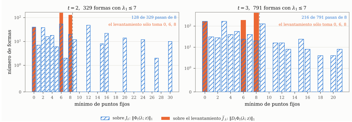
Figura 12. Lo que el levantamiento le hace al recuento. Por el Lema 6.6 una involución de la especie requerida deja al menos \|\Phi_t(\lambda; z)\|_1 puntos fijos sobre J_\lambda y al menos \|D_t\Phi_t(\lambda; z)\|_1 sobre \hat{J}_\lambda ; las dos se dibujan como distribuciones sobre las mismas formas, en recuento logarítmico. La línea discontinua está en ocho, que es el máximo de monomios que el Lema 4.3 puede dar, así que lo que hay que leer es la extensión horizontal y no la forma de ninguno de los dos histogramas: el requisito sin levantar pasa de la línea —hasta 30 en t=2 y 21 en t=3 , en 128 y 216 de las formas— y el levantado no puede, tomando sólo los valores 0, 6 y 8. Para \Phi_t \neq 0 el mínimo levantado es 6 u 8, y la Proposición 6.10 dice que es exactamente 2|\mathcal{U}(\lambda)| ; el valor 0 corresponde a los casos de anulación, donde esa proposición no se aplica. Sobre el lugar no nulo el levantamiento no mueve el requisito: lo aplasta exactamente sobre el recuento de Laplace. El azul va hueco sobre el naranja para que los dos se vean donde se solapan, y la población excluye la partición vacía, como hace la corrida archivada. Calculada por anc/fig_lift.py , que reconstruye J_\lambda desde (20) y no comparte código con los guiones de la §9.
