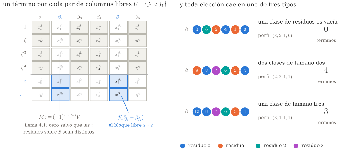
Figura 8. La arquitectura de la demostración, dibujada con t = 4 , N = 6 . Izquierda: el determinante \det(x_i^{\beta_j}) desarrollado por las t filas congeladas. Cada elección de las dos columnas U = \{j_1 < j_2\} que se dejan a las filas libres z, z^{-1} deja un menor t \times t M_S sobre las columnas complementarias, que por el Lema 4.1 vale \pm V o cero, por el bloque 2 \times 2 f(\beta_{j_1} - \beta_{j_2}) . Derecha: por el recuento del exceso dos (3) sólo hay tres perfiles de residuos, uno por fila, cada uno sobre un beta-conjunto que lo realiza; el número de la derecha es cuántas elecciones de U sobreviven, contado y no afirmado — 0, 4 y 3, que es la tricotomía sobre la que se organiza la sección. El color es la clase de residuos. Calculada por anc/fig_proof.py .
