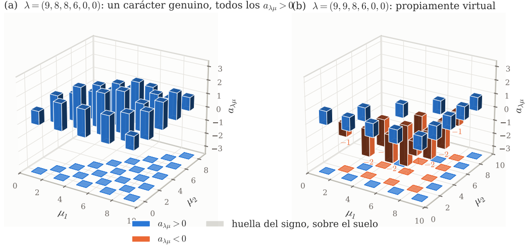
Figura 20. Por qué un solo par recíproco no es lo típico, en r = 2 : la expansión \Psi_r(\lambda) = \sum_{\mu} a_{\lambda\mu} sp_{\mu}(z) sobre los pesos dominantes de Sp(4) . Las dos formas difieren en una sola casilla. Para \lambda = (9, 8, 8, 6, 0, 0) todo a_{\lambda\mu} es positivo: el objeto es un carácter genuino, como lo es para toda \lambda cuando r = 1 , donde el Teorema 3.1 lo escribe como producto de tres caracteres de \mathfrak{sl}_2 . Para \lambda = (9, 9, 8, 6, 0, 0) la expansión tiene 12 coeficientes positivos y 10 negativos, siendo el más negativo -3 : es genuinamente virtual, que es el fenómeno que recoge la Observación 8.12 y la razón de que un cálculo en el extremo deje de ser un test exacto pasado un par. Los dos paneles comparten la escala vertical, y los cuadrados planos del suelo repiten el signo de cada coeficiente, porque un coeficiente -1 es invisible al lado de uno +3 . Calculada por anc/fig_v2.py .
