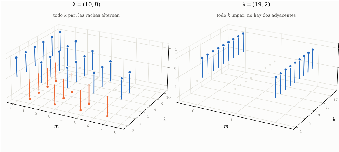
Figura 11. La Proposición 6.4, dibujada. Para cada k las \nu admisibles son la única familia (m+k, m) , y se representa \sigma_m = s_{\lambda/(m+k,m)}(1, -1) frente a m y k ; los puntos grises son los ceros. Toda barra tiene altura exactamente \pm 1 , que es la parte (i): los términos forman un conjunto, luego la cancelación que pide la enumeración es un emparejamiento y no algo con multiplicidad. A la izquierda todo k es par y el color alterna a lo largo de cada racha, que es la parte (iii) y lo que hace que m \leftrightarrow m+1 invierta el signo; donde una racha acaba, la acaba un cero. A la derecha todo k es impar y no hay dos términos no nulos contiguos, que es la parte (ii): las rachas tienen longitud uno y no hay nada que cancelar.
