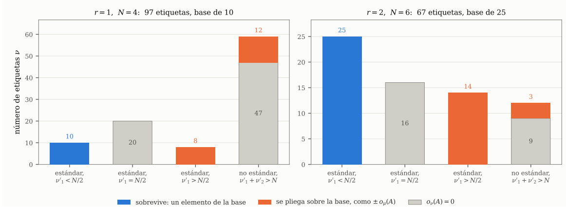
Figura 15. La reducción del Lema 8.9, dibujada. Cada etiqueta \nu que aparece en s_\lambda = \sum_\nu c_\nu o_\nu se coloca en una de cuatro clases y se calcula su valor o_\nu(A) . Las etiquetas autoasociadas se anulan, todas ellas; las estándar con \nu'_1 > N/2 se pliegan sobre la base como \pm o_\mu(A) ; las no estándar o se anulan o se pliegan sobre un único elemento de la base con coeficiente \pm 1 . Por (26) estas tres son las reglas de modificación simplécticas disfrazadas, con las clases cortadas por \ell(\nu) frente al rango r ; la figura se calculó antes de advertirlo y se deja tal cual. Todo aterrizza en la base independiente \{o_\mu(A) : \ell(\mu) \leq r\} , que es lo que convierte la anulación en la condición finita (27). Las alturas de las barras son recuentos de etiquetas sobre el rango en que se calculó cada panel, menor que el de la fila correspondiente de la §9; lo que la imagen cuenta es la clasificación, no el recuento.
