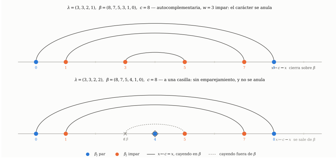
Figura 14. Por qué la autocomplementariedad mata el carácter. Al desarrollar por las dos filas congeladas quedan términos indexados por pares (e, o) con e \in E , o \in O , y la reflexión x \mapsto c - x actúa sobre ellos. Arriba, una forma autocomplementaria de anchura impar: todo arco cae dentro de \beta y une entradas de igual paridad, porque c es par. Abajo, la misma forma con una caja movida: el arco 5 \mapsto 3 se sale de \beta , así que no hay emparejamiento y nada se cancela. El rombo marca el punto fijo de la reflexión, que no puede darse dentro de un par de paridades opuestas —y ésa es la razón de que la involución sea libre.
