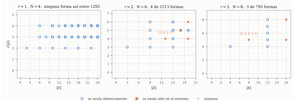
Figura 16. Dónde deja de ser típico un solo par recíproco. Cada partición con a lo sumo N partes es un punto en (|\lambda|, \ell(\lambda)) ; la clase dibujada con estrella es la que se anula en el extremo z_i = 1 sin anularse idénticamente, y es todo el contenido de la imagen; cada panel nombra a su miembro más pequeño y la Observación 8.12 enumera los demás. Los paneles cubren |\lambda| \leq 24, 20 y 16 respectivamente. En r = 1 la clase está vacía sobre las 1292 formas del rango, porque allí el objeto es \pm un carácter genuino y su valor en la identidad es una dimensión. A partir de r = 2 aparecen ejemplos genuinamente virtuales y la clase deja de estar vacía —no que toda forma lo sea: el Cuadro 2 cuenta las dos cosas—. Véase la Observación 8.12.
