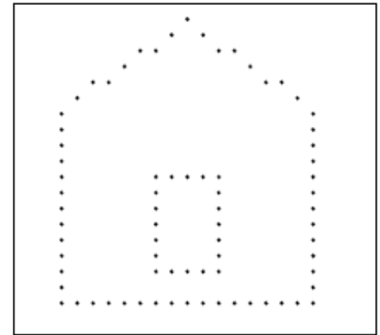
Rastergrafik: Pixelmatrix
