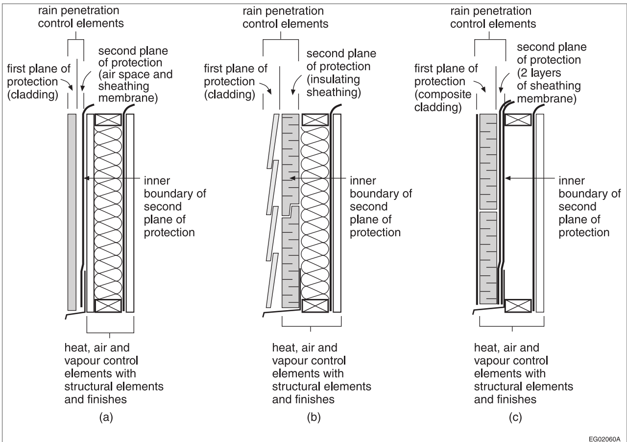
Figure A-9.27.2.
