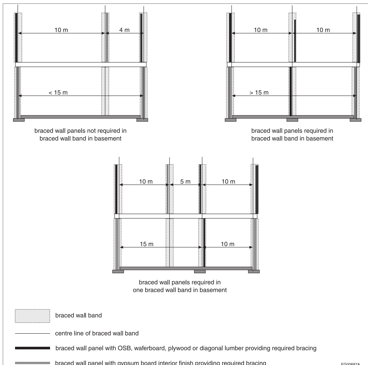
Figure A-9.23.13.5(2)
