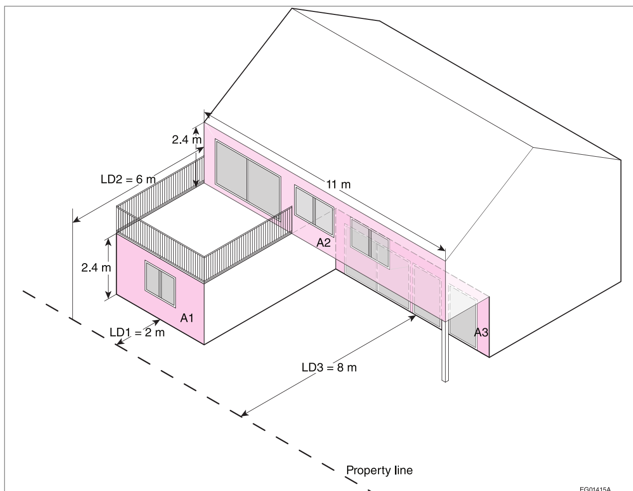
Figure A-9.10.15.4.(2)-D
