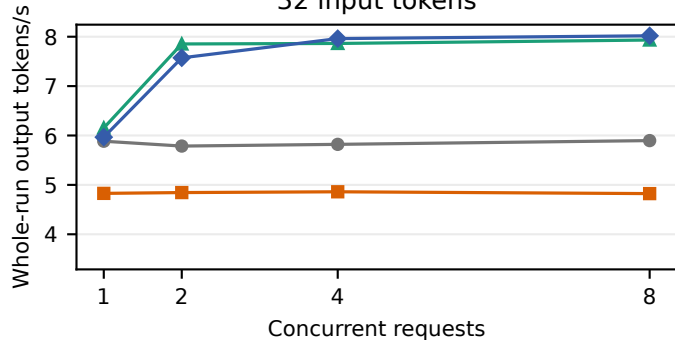
32 input tokens
