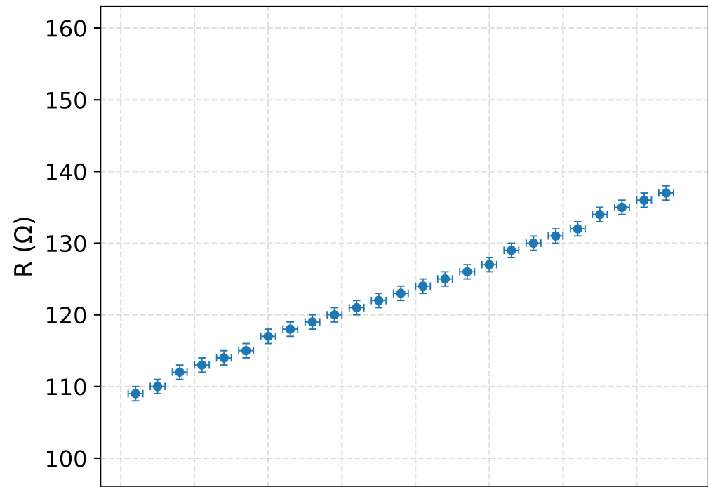
Platyna (Pt) – Ogrzewanie
