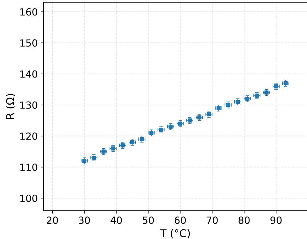
Platyna (Pt) – Chłodzenie
