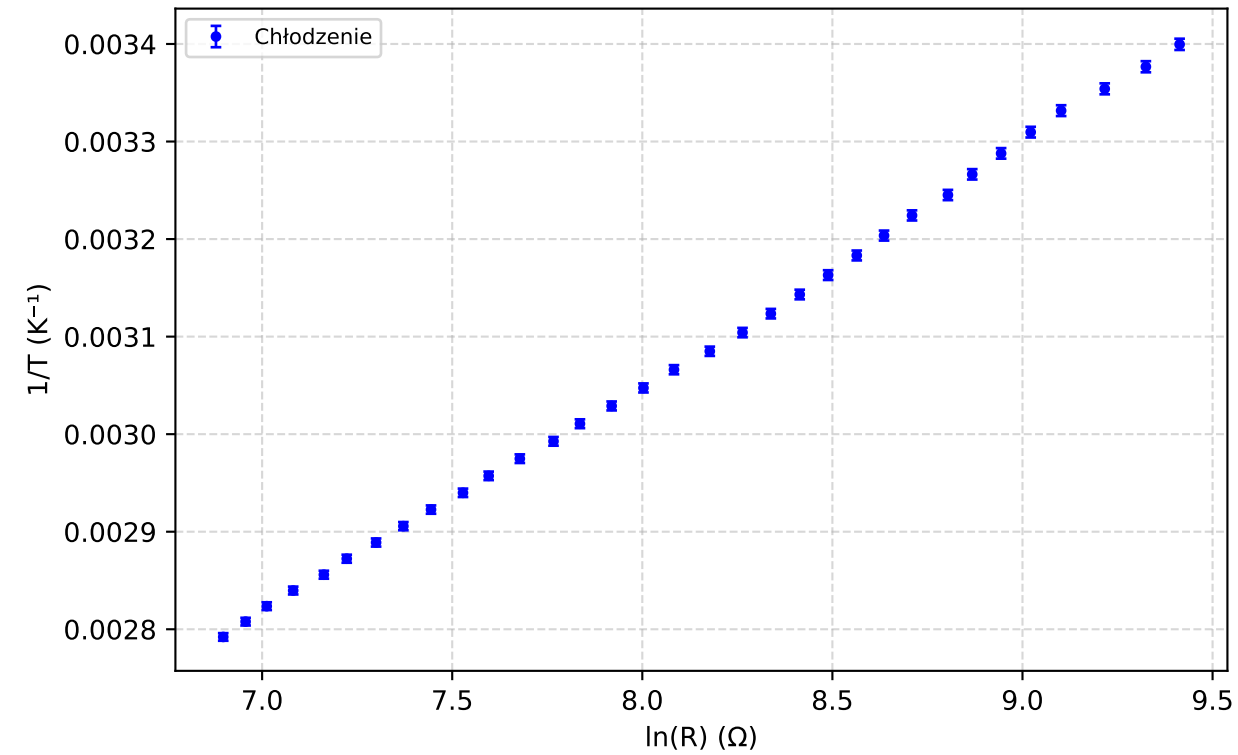
Termistor — Chłodzenie
