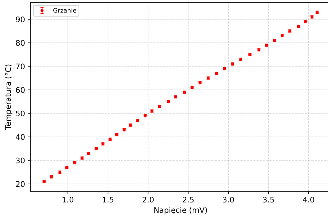
Termopara — Grzanie
