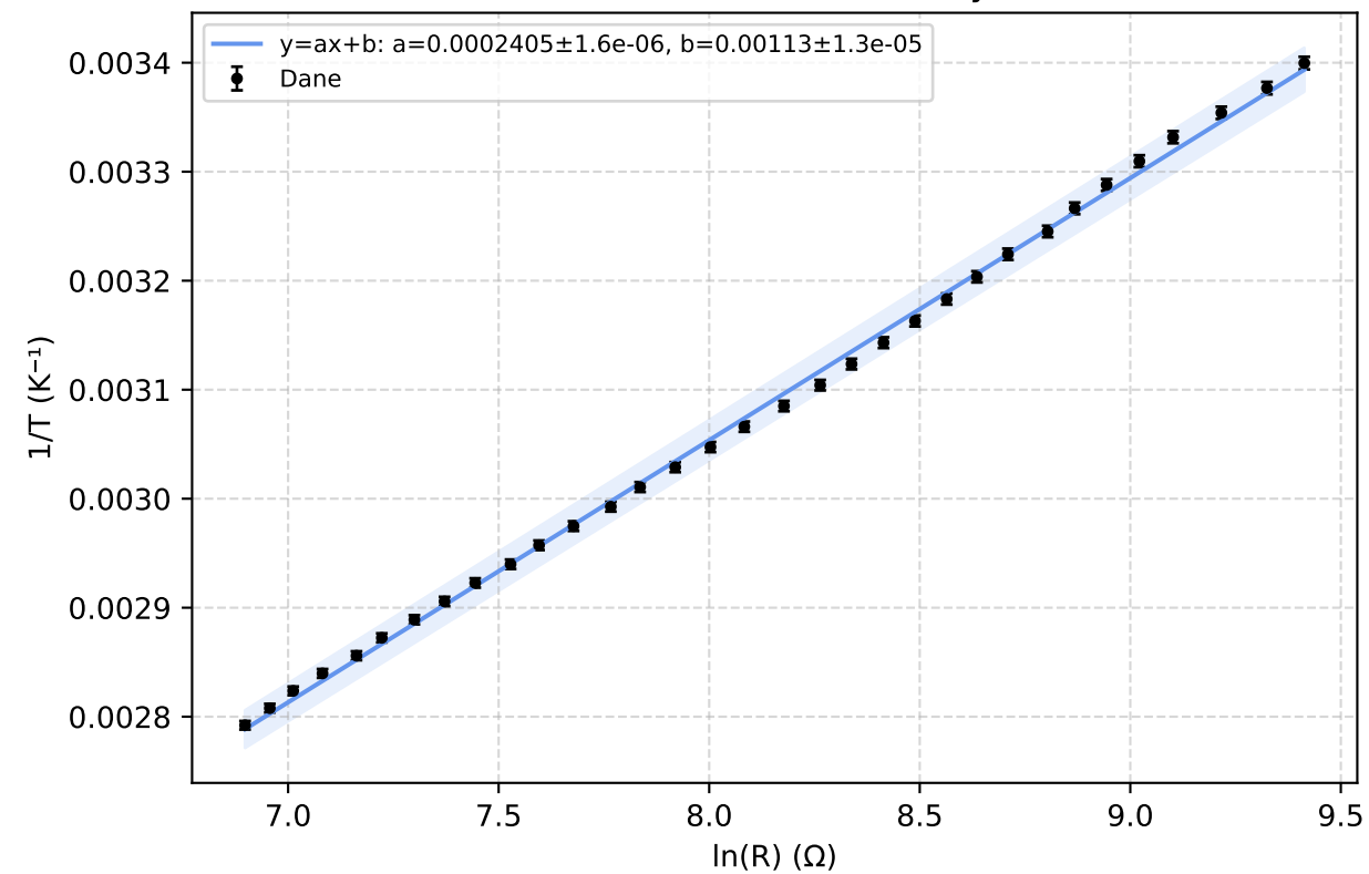
Termistor — Chłodzenie (wszystkie)
