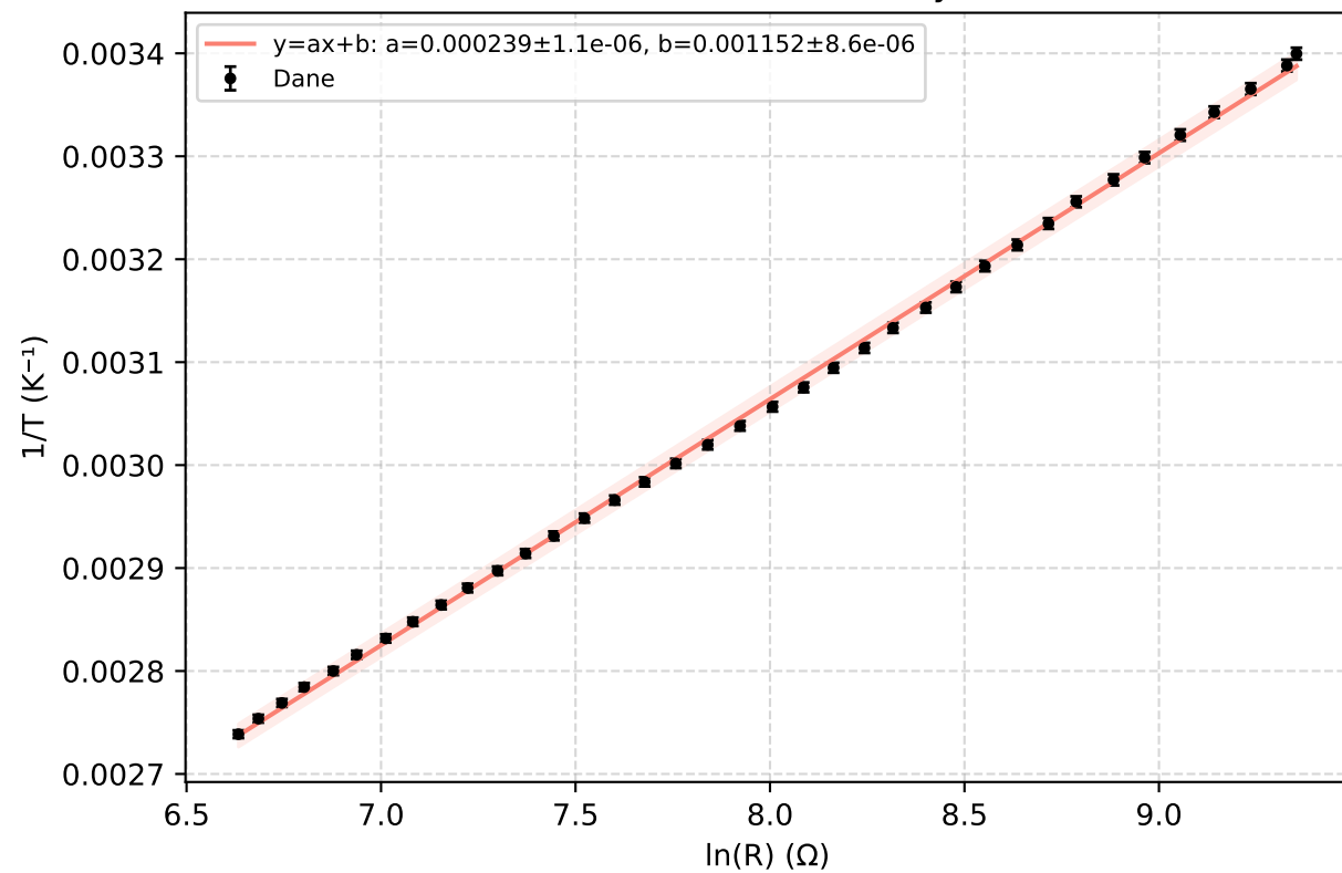
Termistor — Łączone
