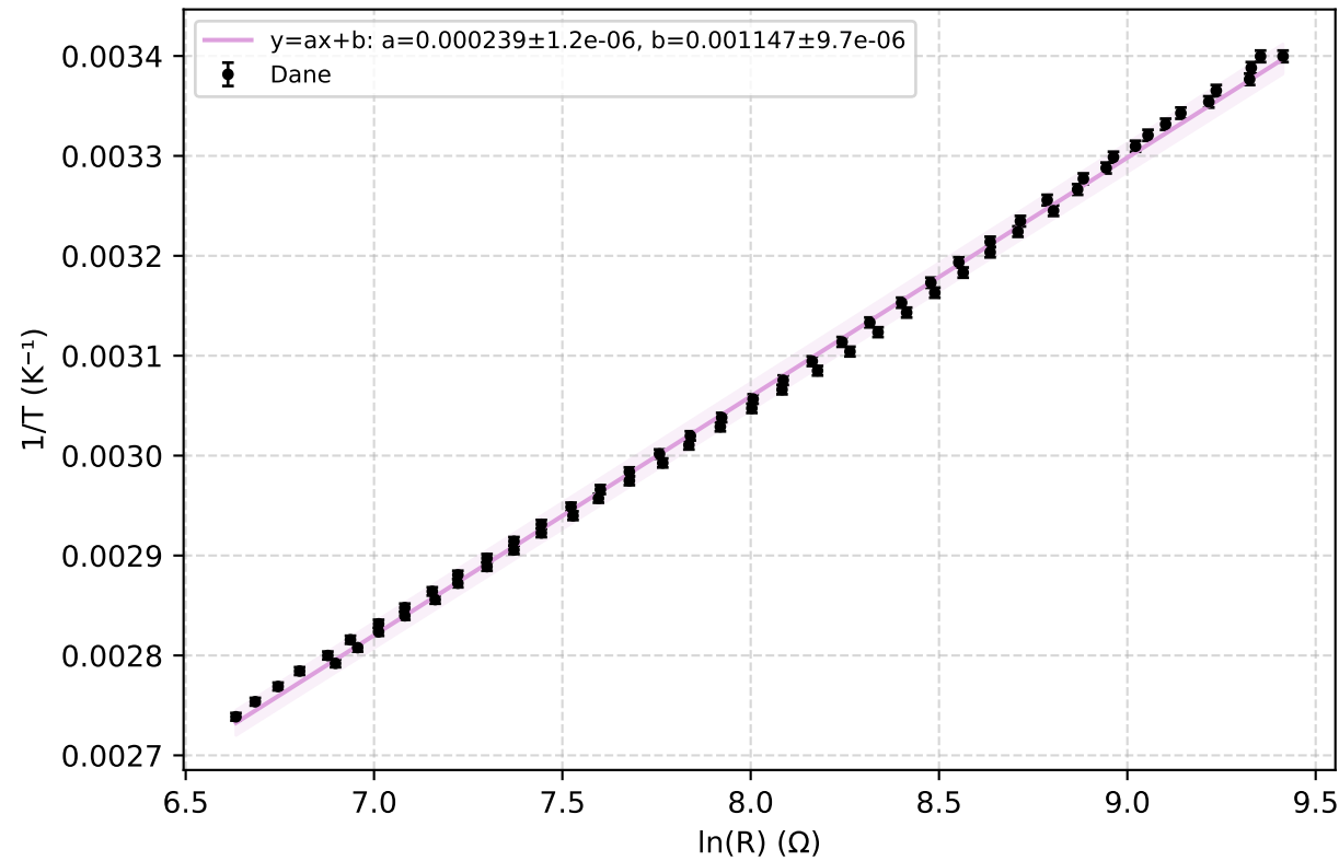
Termistor — Łączone
