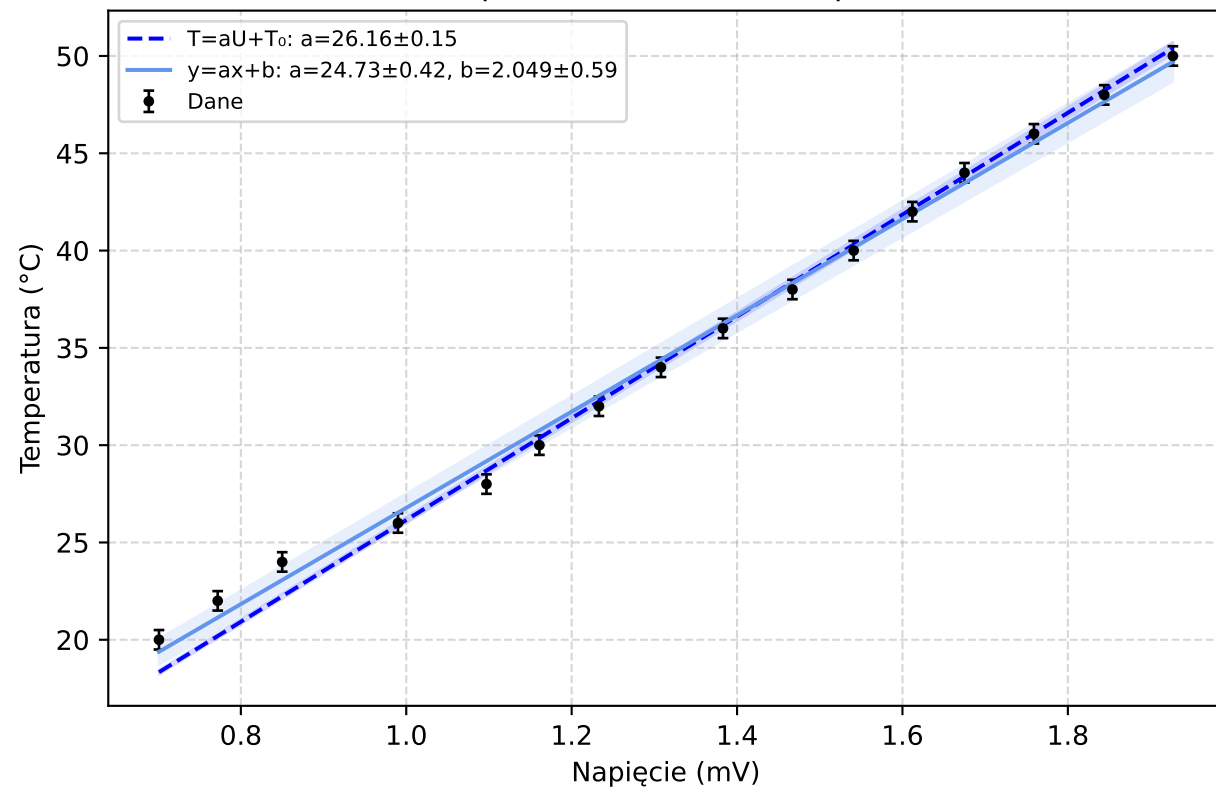
Termopara — Chłodzenie 1. połowa
