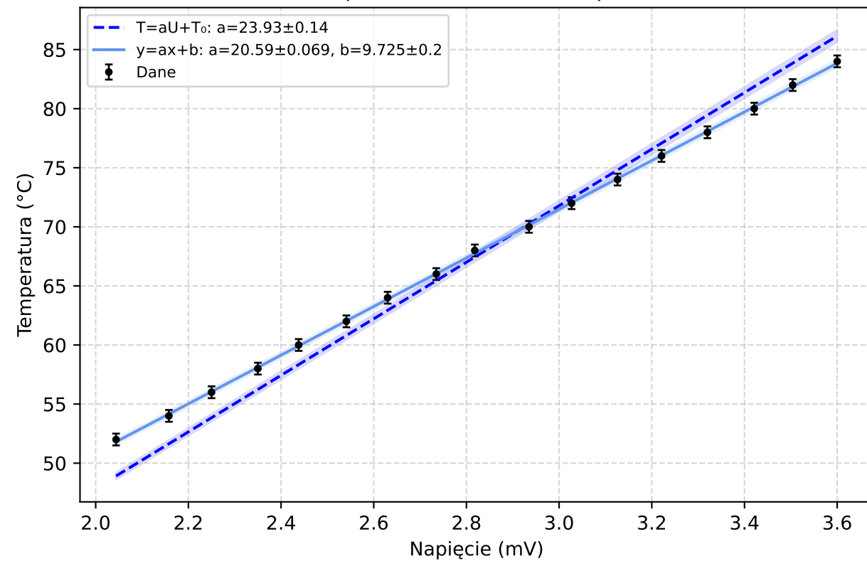
Termopara — Chłodzenie 2. połowa
