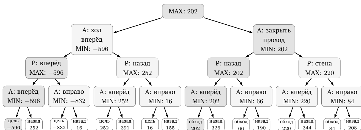
Рис. 8 — Фрагмент дерева Минимакса
