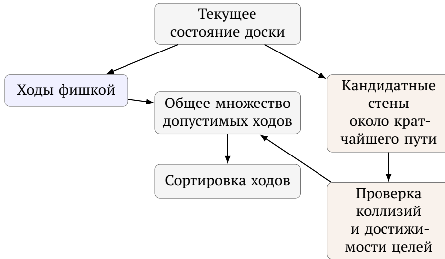
Рис. 4 — Формирование множества допустимых ходов
