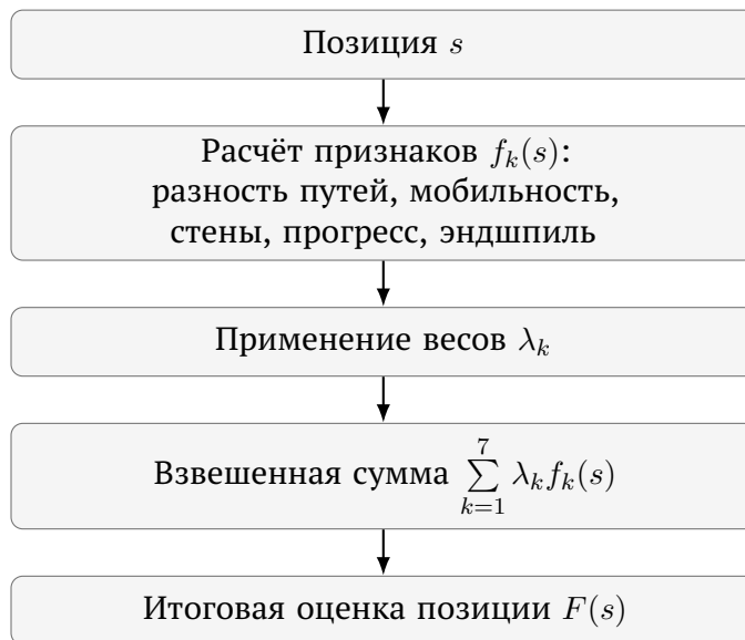
Рис. 6 — Вычисление оценки игровой позиции
