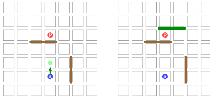
Рис. 7 — Два варианта хода, сравниваемые функцией оценки
