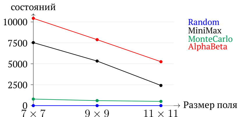
Рис. 11 — Среднее число просмотренных состояний при изменении размера поля
