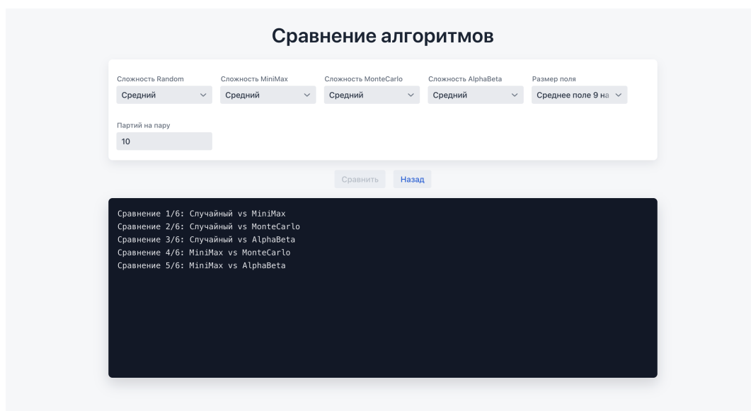
Рис. 15 — Экран сравнения алгоритмов
