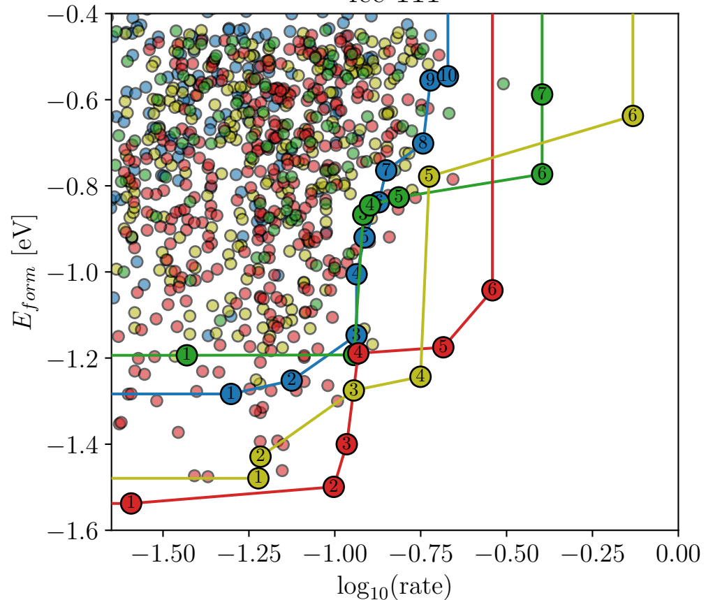
fcc-111
