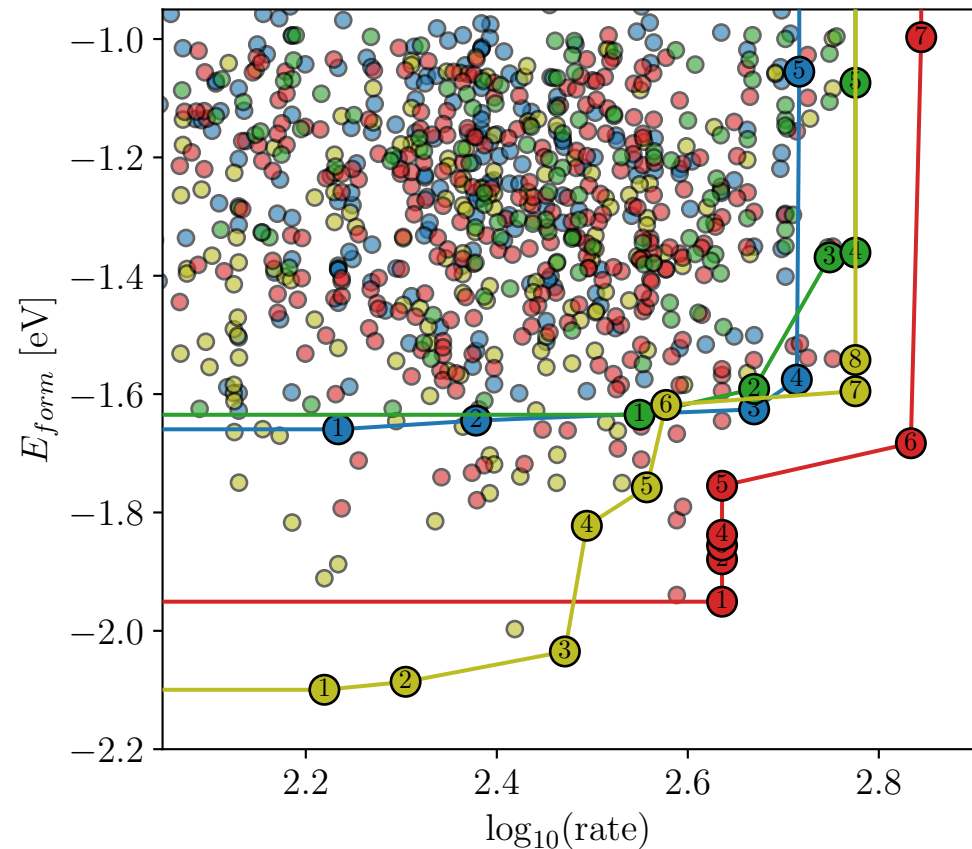
fcc-100
