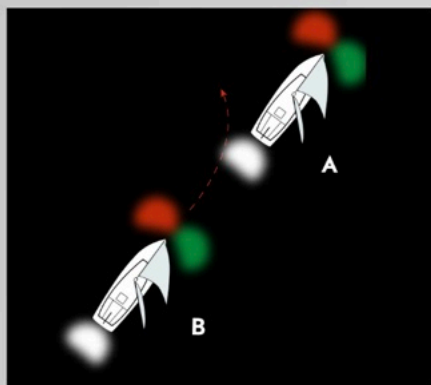
Nähert sich ein Fahrzeug einem anderen im Bereich des Hecklichts, muss es ausweichen. A sieht von B rot-grünes Licht, B von A weißes
