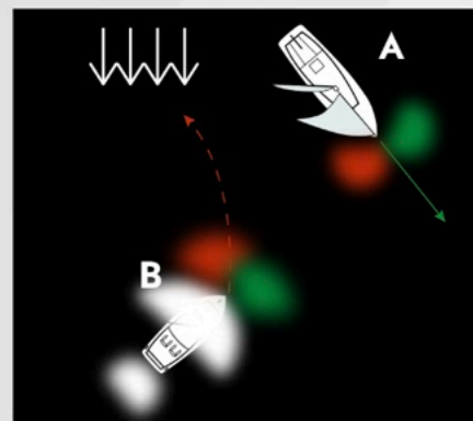
Begegnen sich ein segelndes Boot und ein Motorboot, weicht das Motorboot aus. A sieht von B rotes und weißes Licht, B von A rotes Licht
