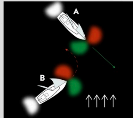
Haben beide den Wind von der gleichen Seite, weicht das luvwärtige Segelboot aus. B sieht von A das grüne, A von B das rote Licht
