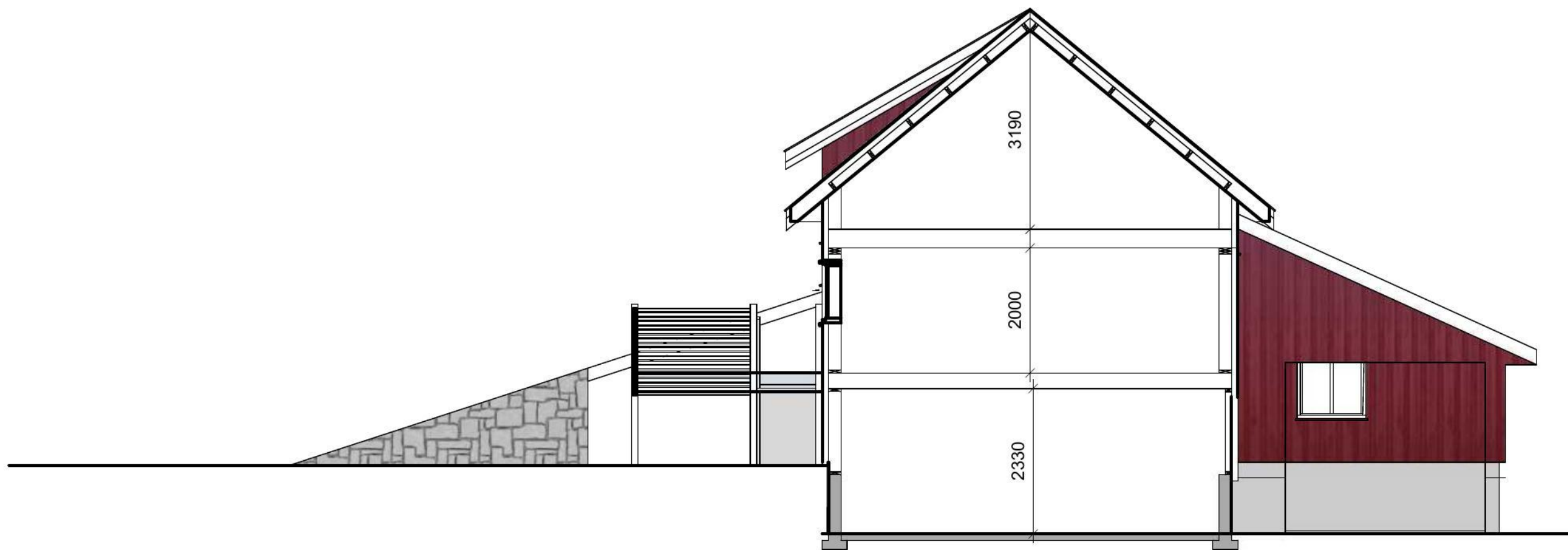
Snitt A-A
