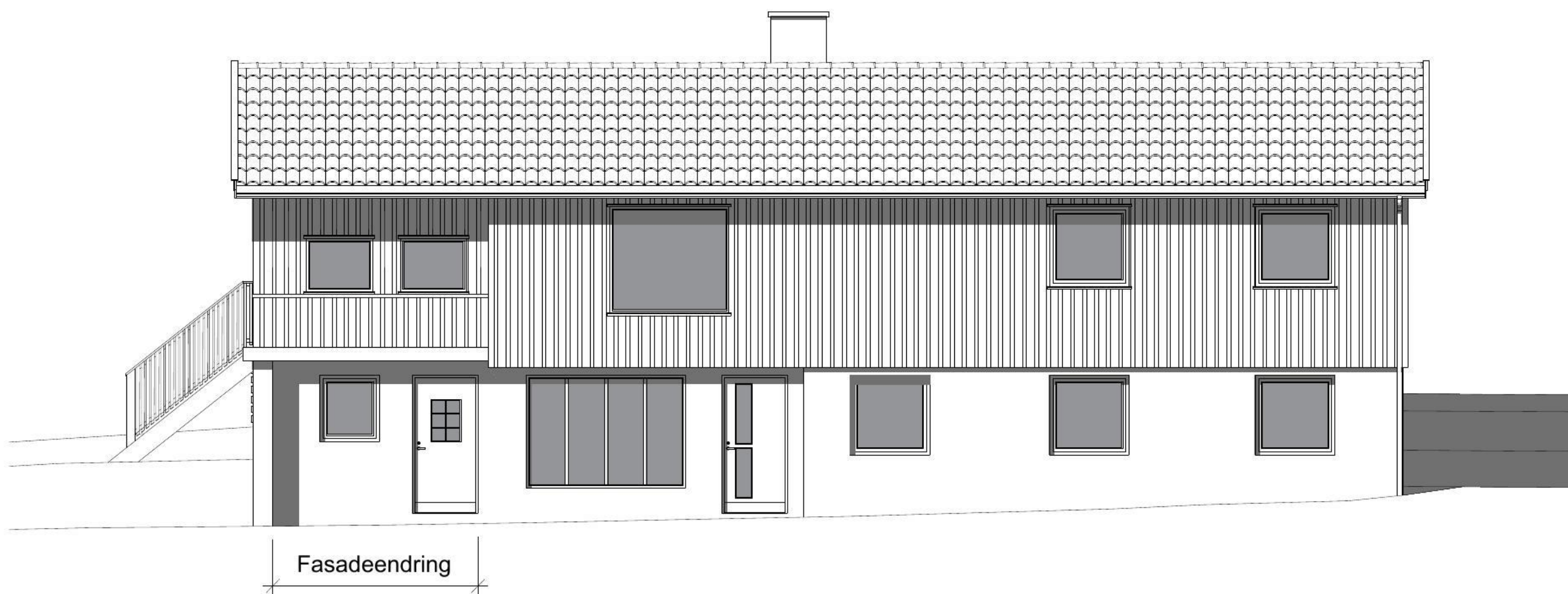
Fasade mot sørøst
