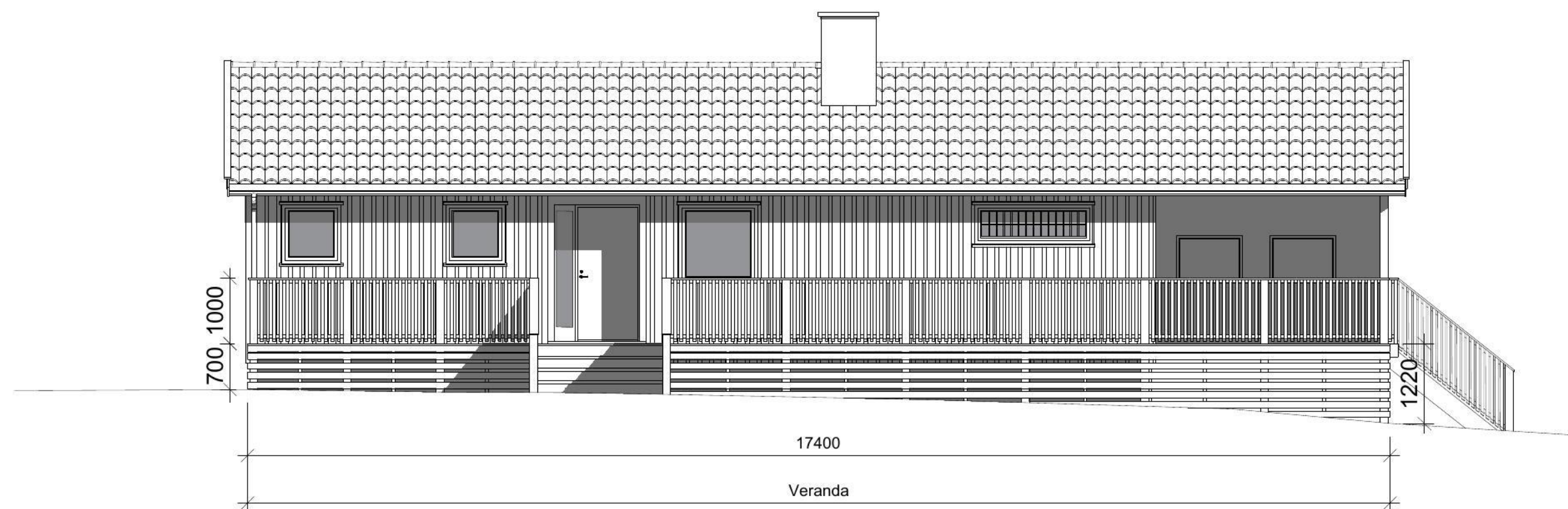
Fasade mot nordvest
