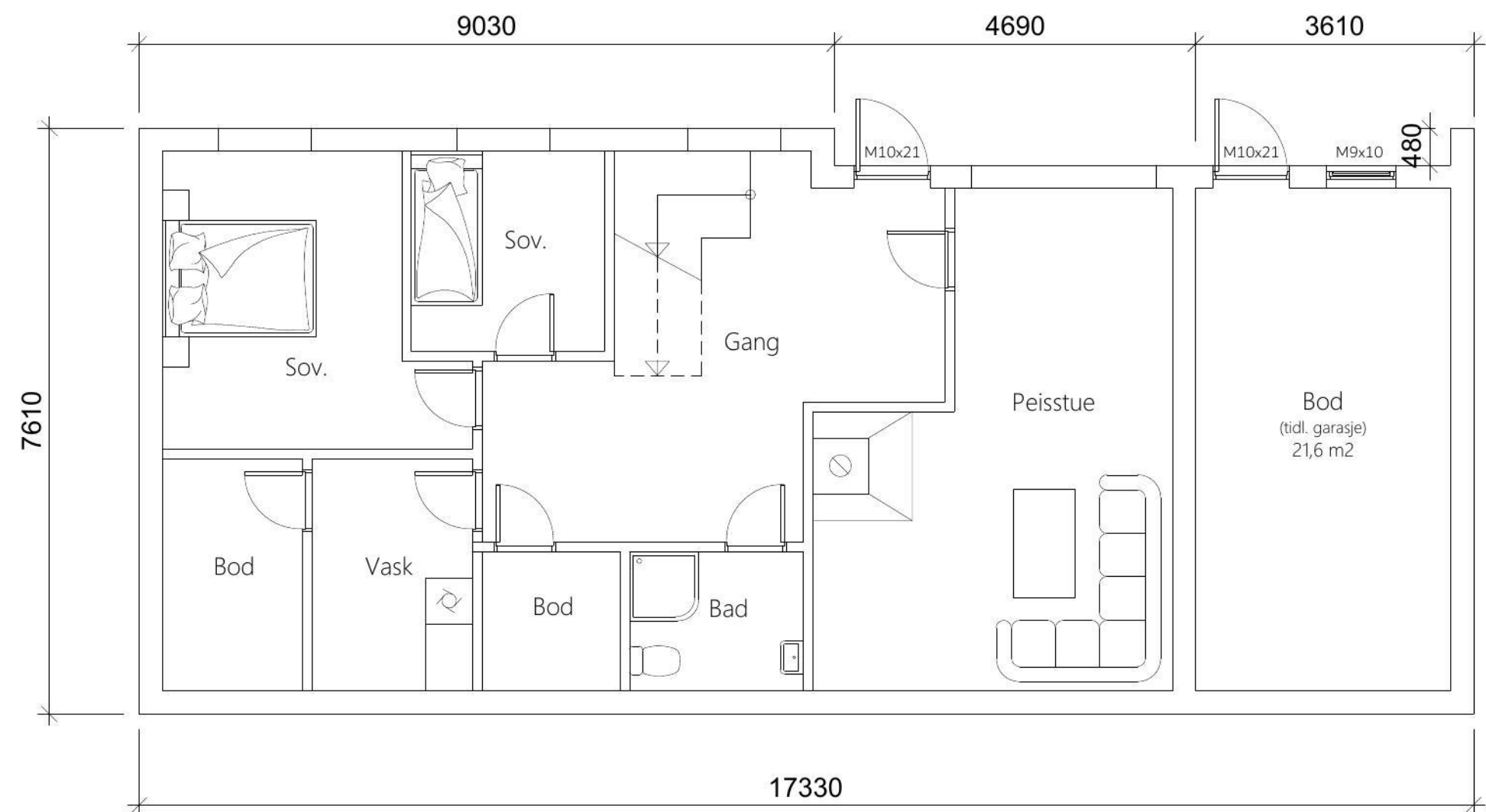
Plan underetasje
