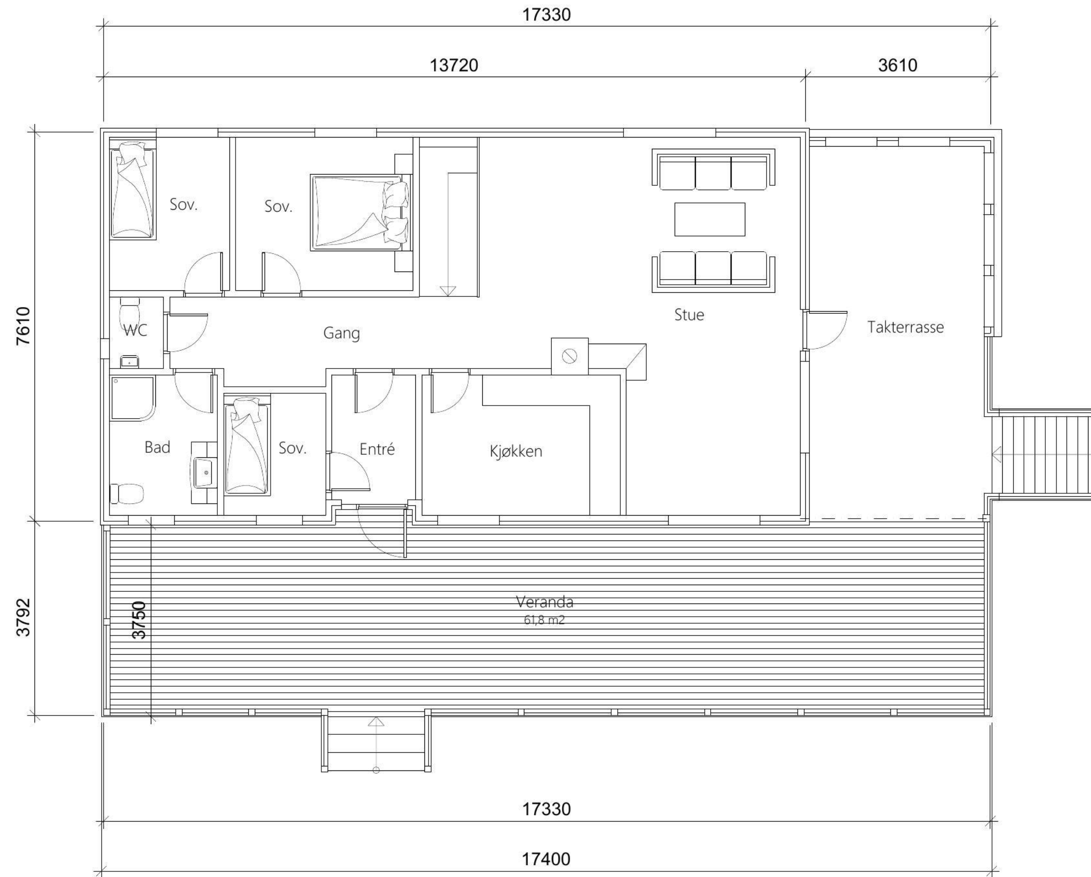
Plan 1. etasje
