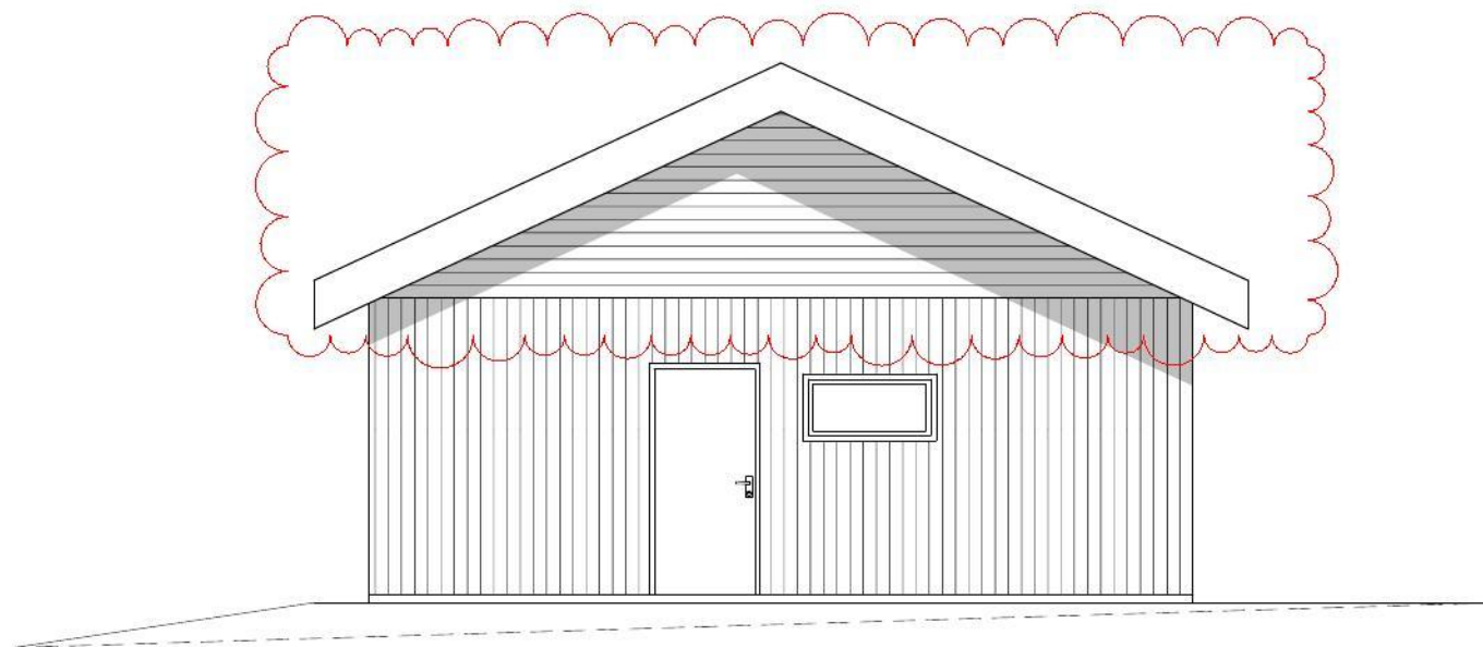
1:100 Fasade Nord
