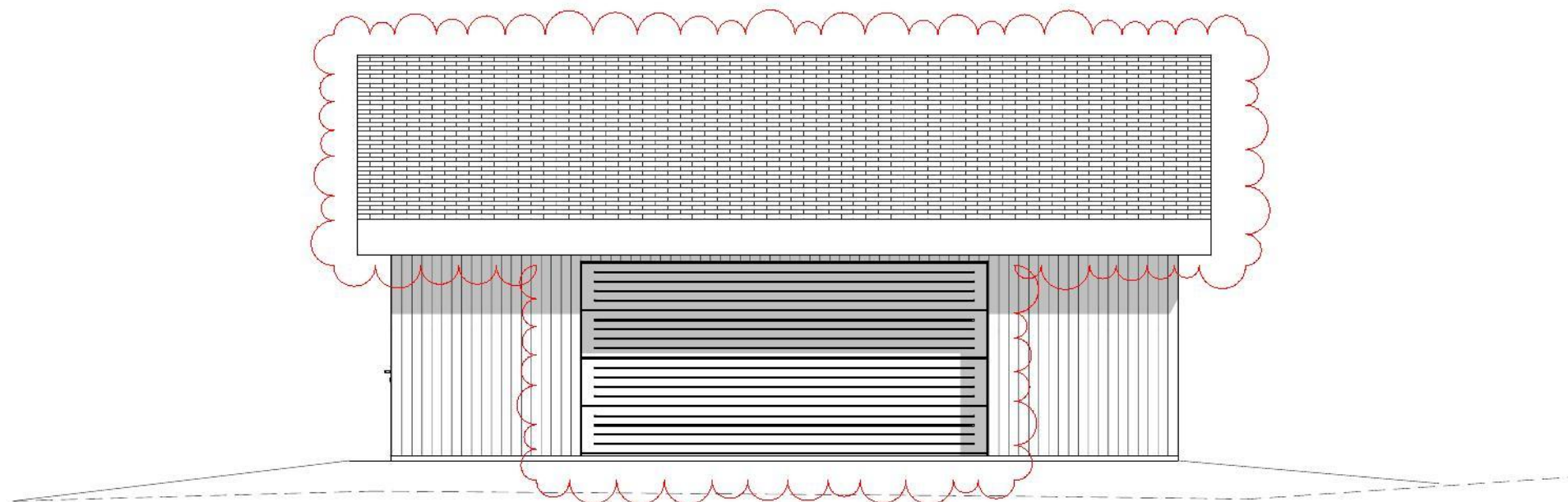
1:100 Fasade Vest
