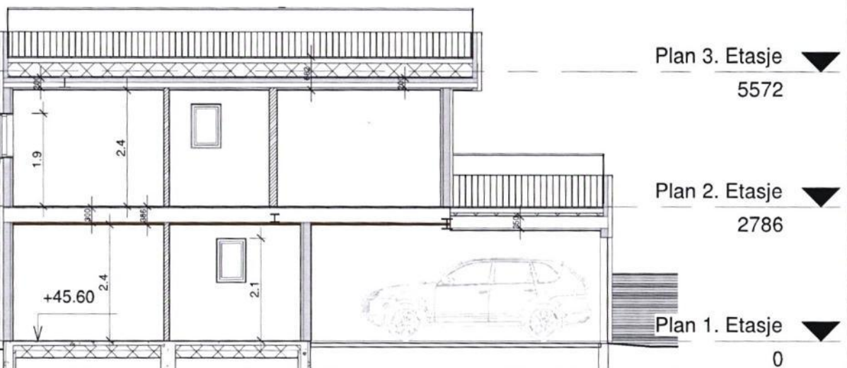
Snitt B-B
