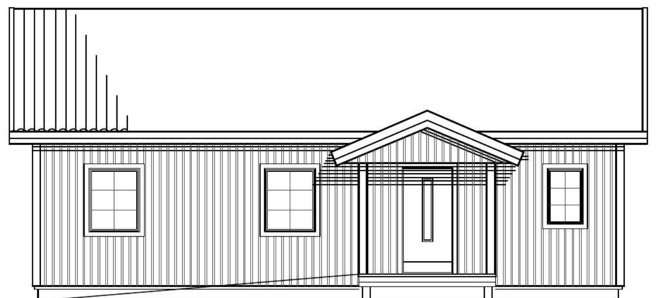
FASADE MOT SYDVEST
