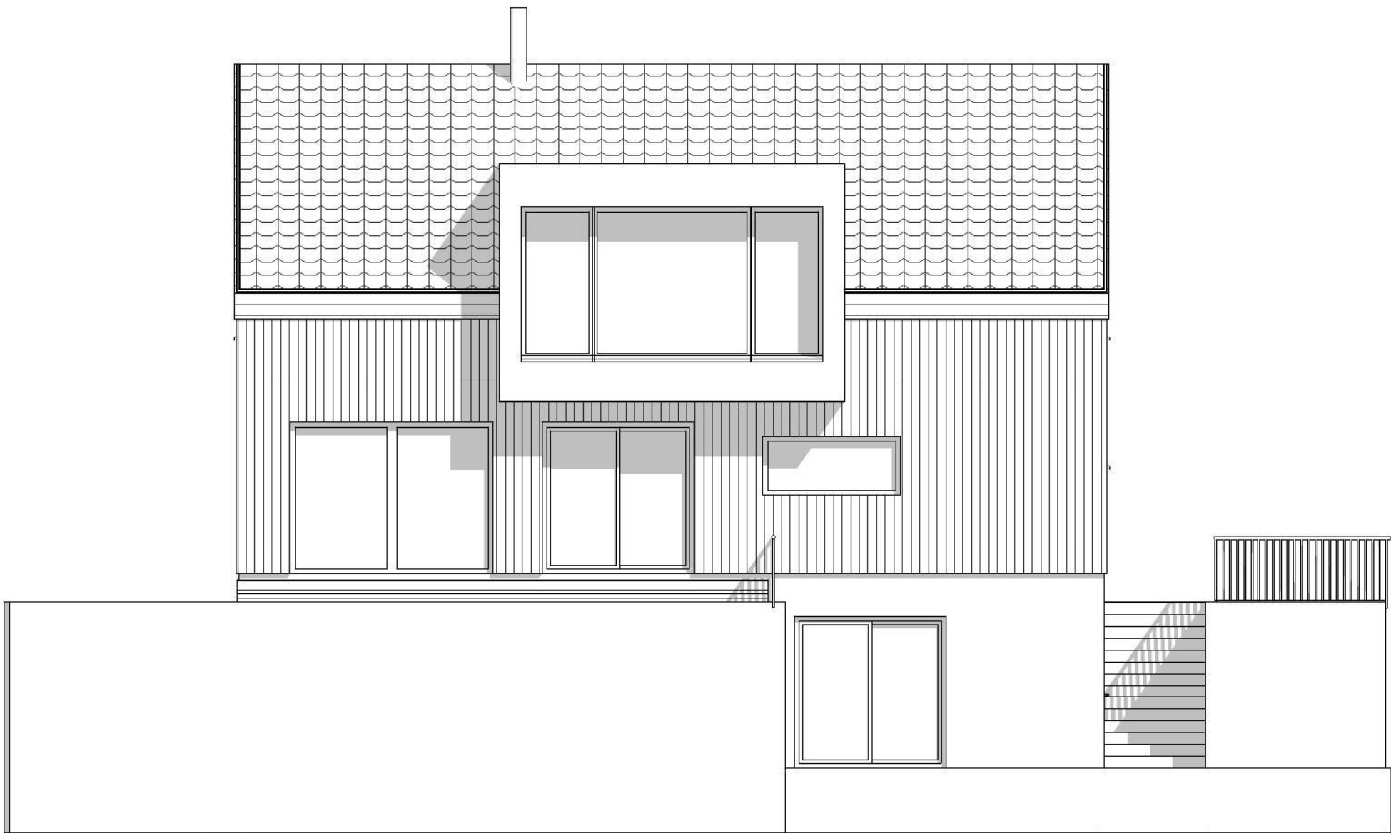
1:100 Fasade Øst
