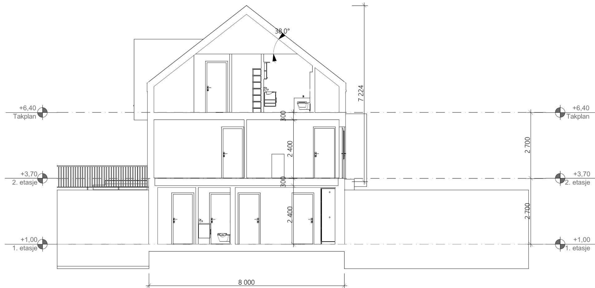
1:100 Snitt A
