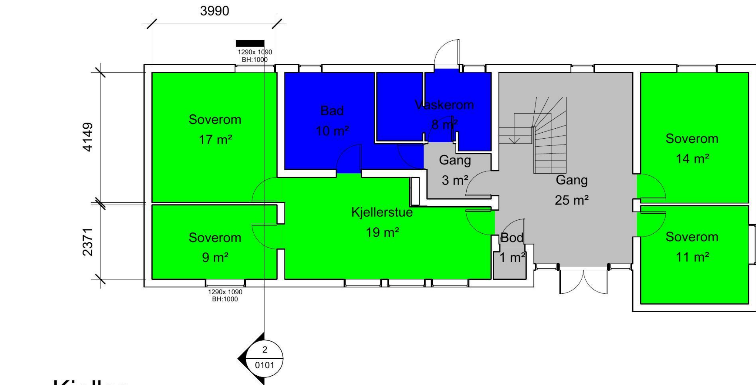
1 Kjeller 1 : 100
