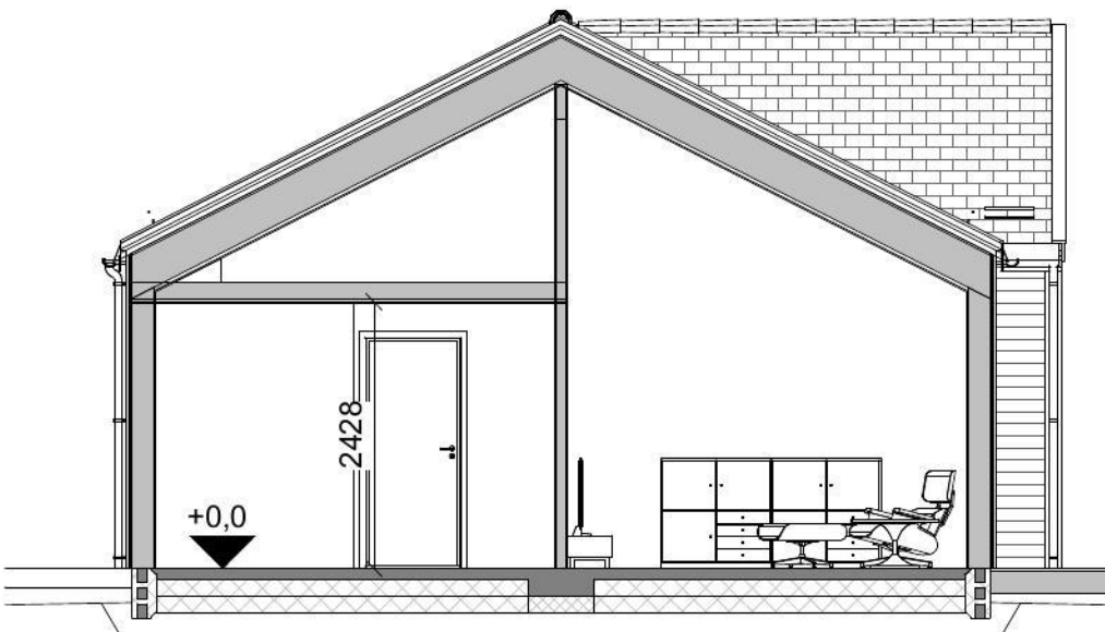
A 1 : 100
