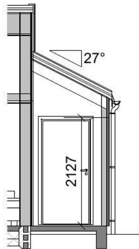
B 1 : 100
