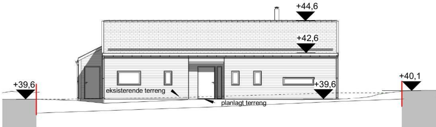
vest 1 : 200
