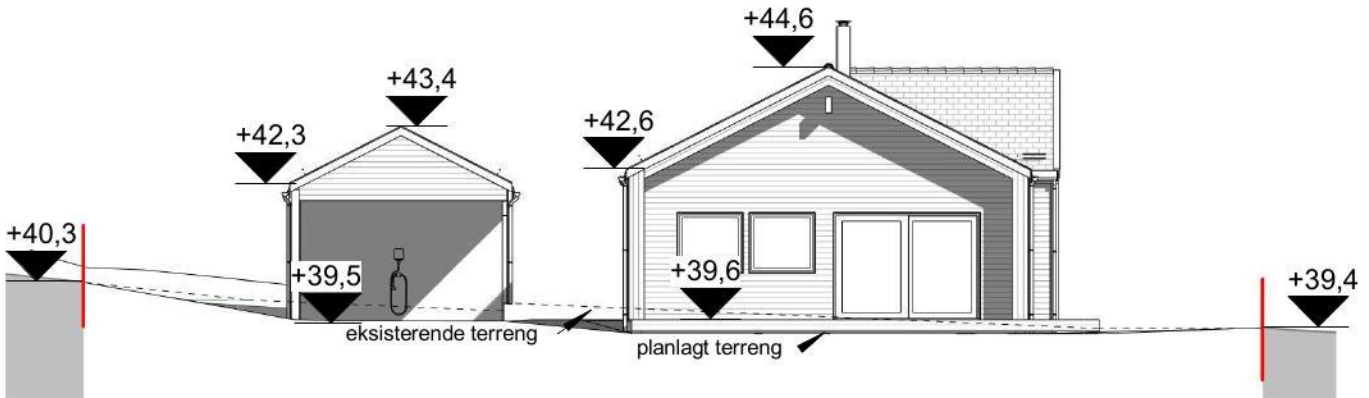
sør 1 : 200
