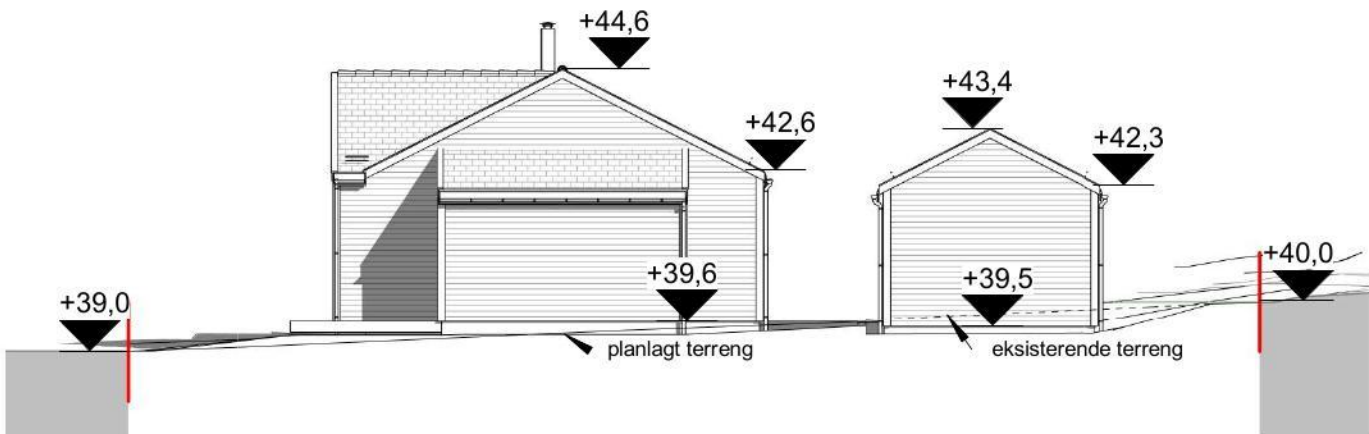
nord 1 : 200
