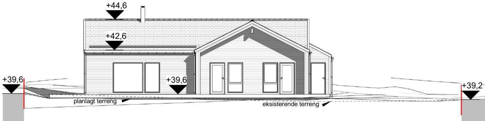
øst 1 : 200
