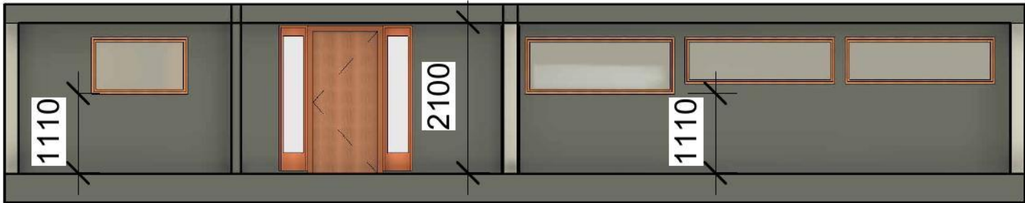
2 Snitt 1 : 100
