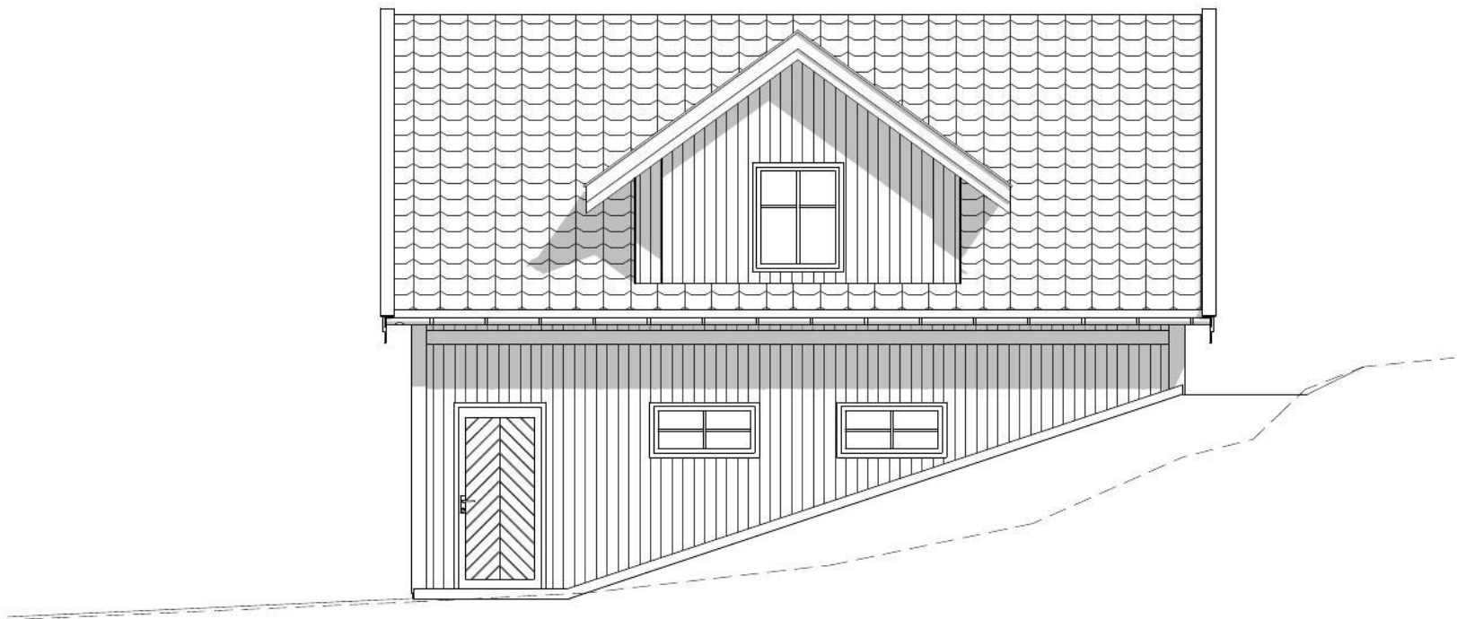
1:100 Fasade Nord
