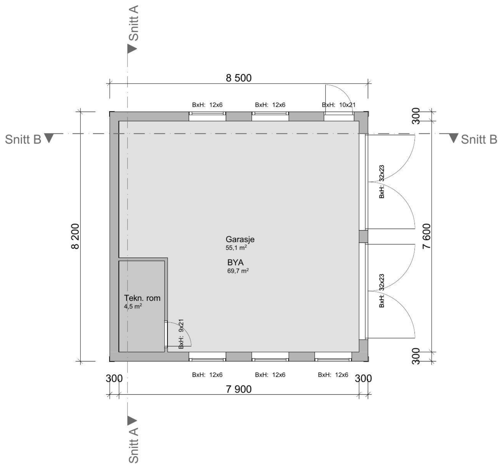
1. Etasje 1:100
