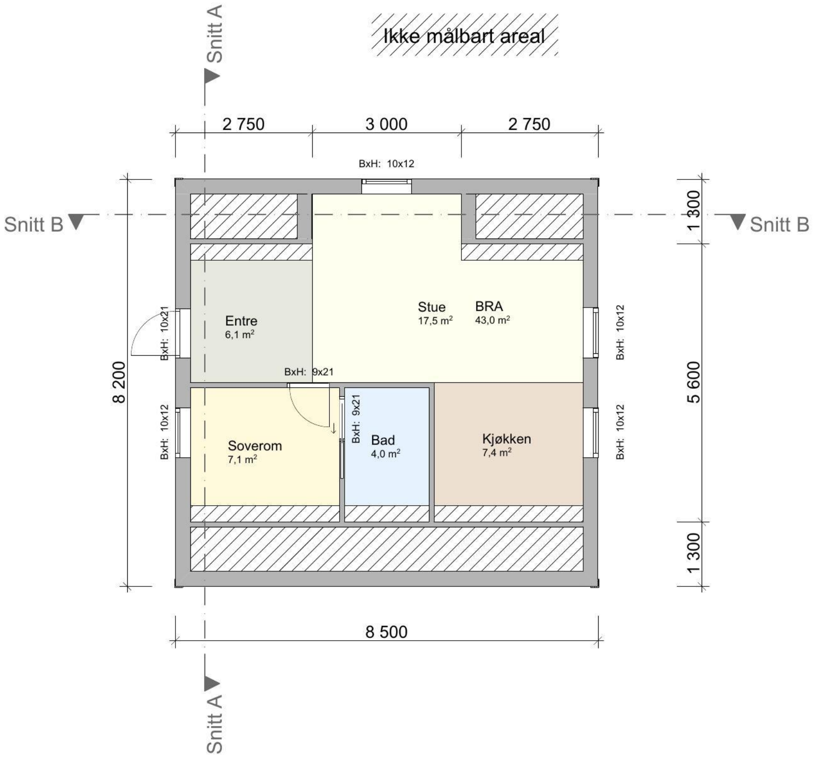
2. Etasje 1:100
