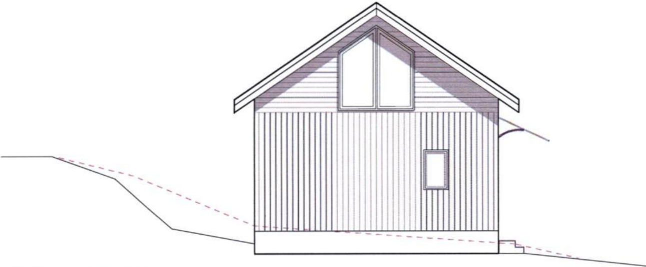
FASADE NORD
