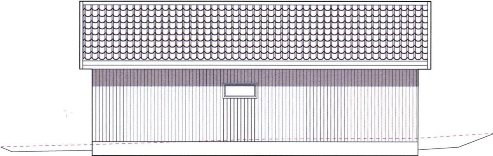
FASADE ØST
