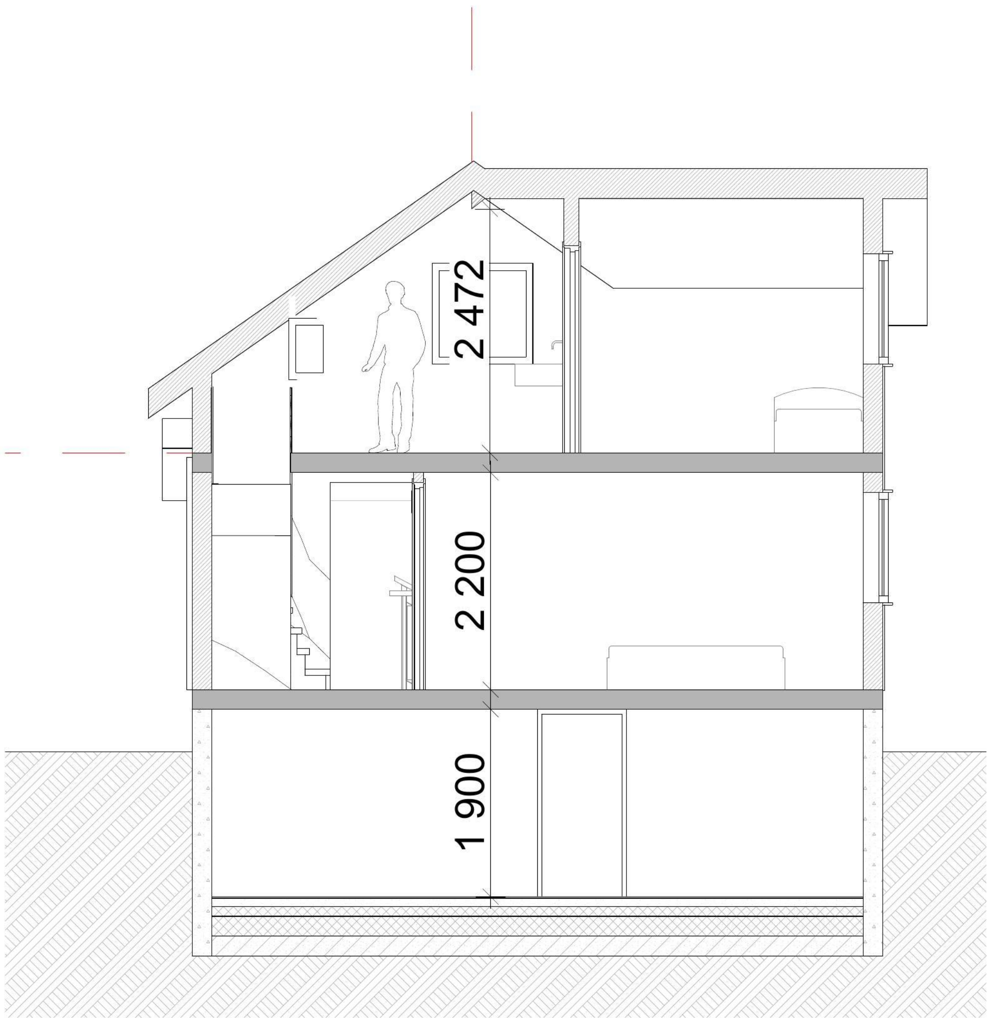
Snitt A
