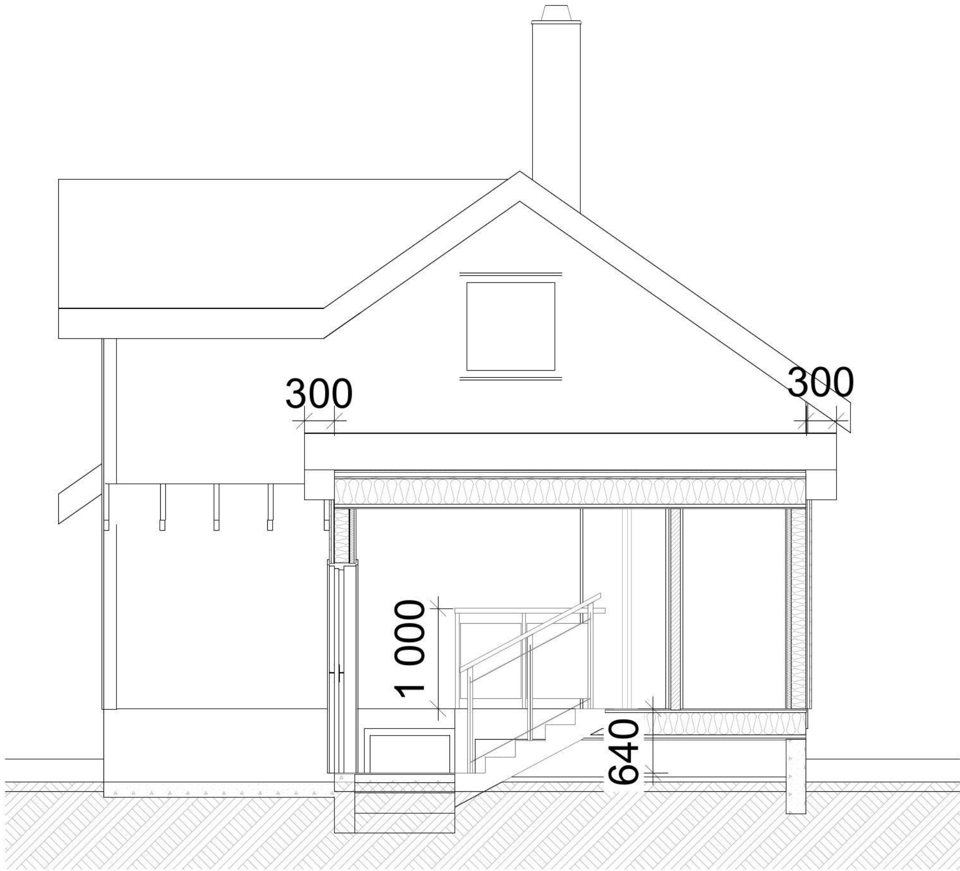
Snitt B
