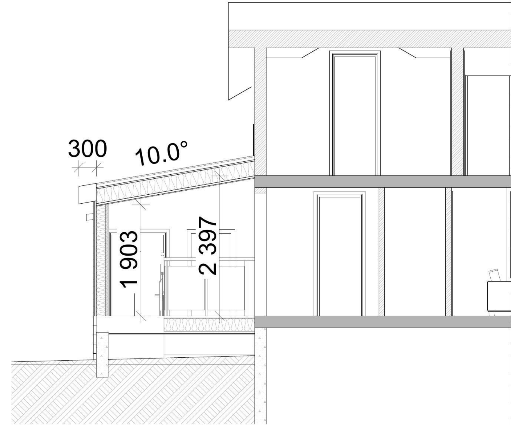
Snitt C
