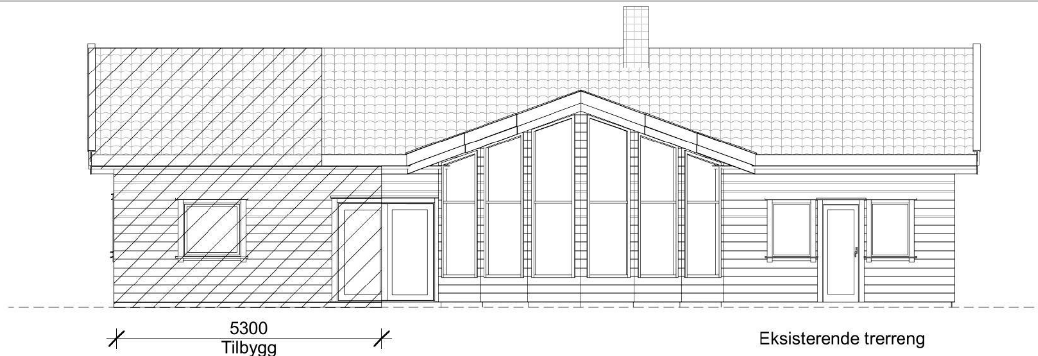
Fasade mot Nord 1 : 100
